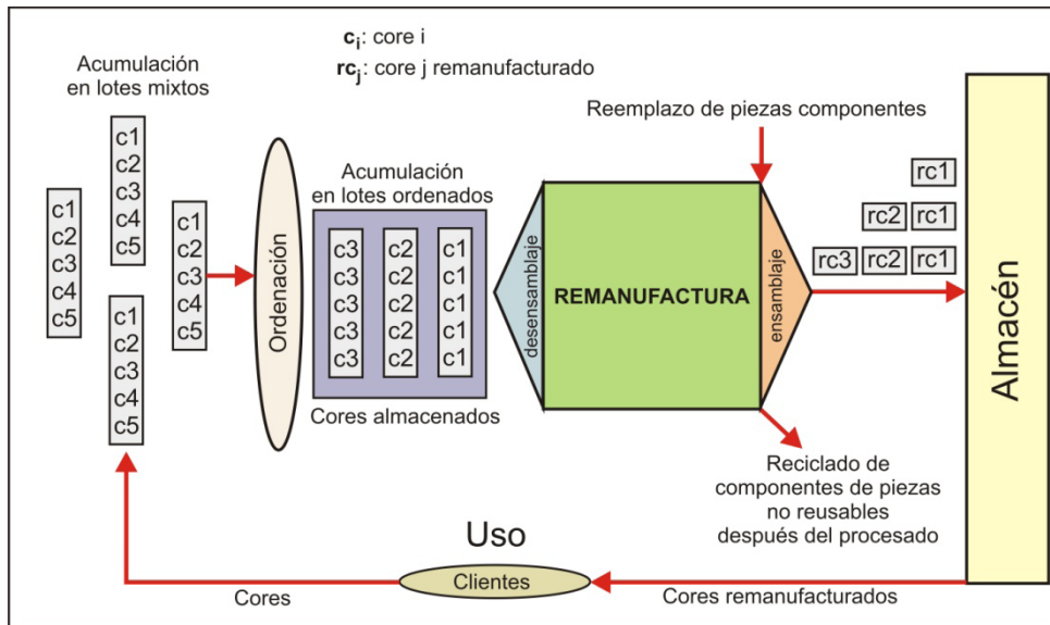
Figura 8. Proceso diseño para la Remanufactura (DfRem).
