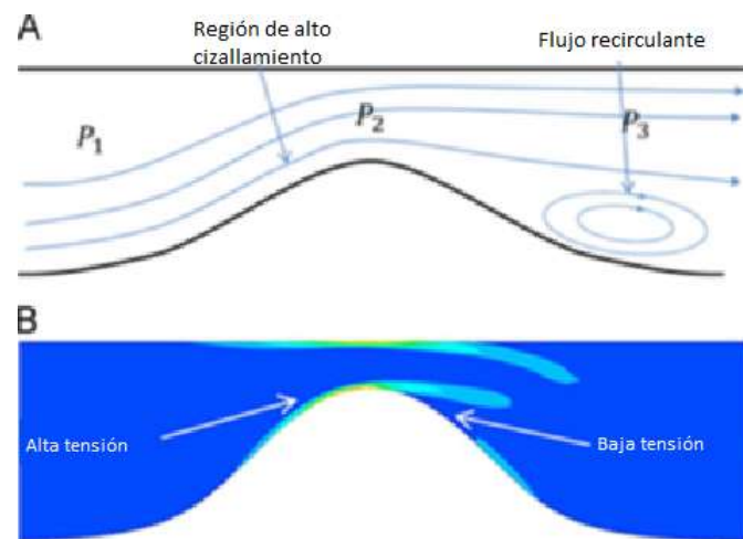
Figura 5. (A) En la ilustración podemos observar las líneas de corriente en un vaso sanguíneo estenotizado. P_1 es la presión de entrada, P_2 la presión en la sección transversal mínima y P_3 es la presión aguas abajo de la constricción. En la ilustración (B) se representa de manera cualitativa la distribución de la tasa de deformación en el sitio de la estenosis de los vasos sanguíneos (Adaptada de Epshtein & Korin, 2017)
