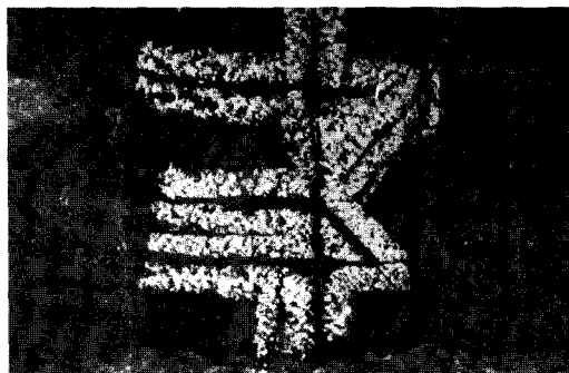
Figura 4 Detalle de montea redibujada con tiza a uno y otro lado de la línea
