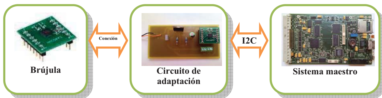
Figura 2. Esquema de conexionado de la brújula.
