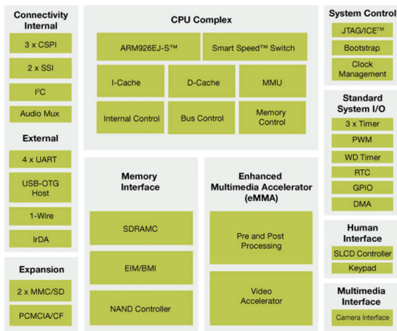
Figura 3. Diagrama de bloques del procesador ARM utilizado.
