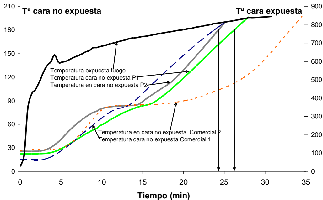
Figura 1. Resistencia al fuego de las placas recicladas frente a dos productos en el mercado (11)
