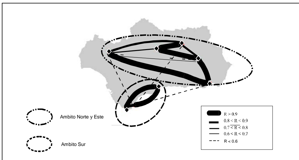
Figura 3. Coeficientes de correlación de Pearson ( r ) calculados entre los coeficientes de variación móviles de los totales anuales de precipitación de los observatorios estudiados
