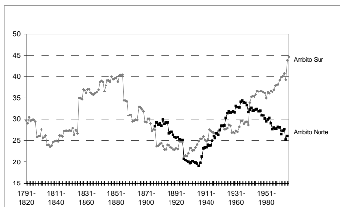
a) Coeficientes de variación móviles de las precipitaciones anuales de las áreas norte y sur de la región.
