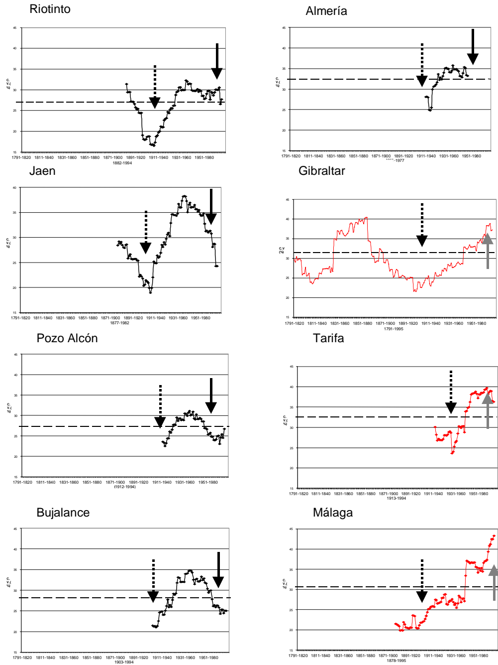
Figura 2. Coeficientes de variación móviles (30 años) de las estaciones seleccionadas
