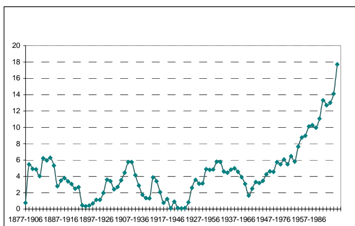
Figura 4. Comportamiento pluviométrico diferencial de las áreas Norte y Sur de la región.
