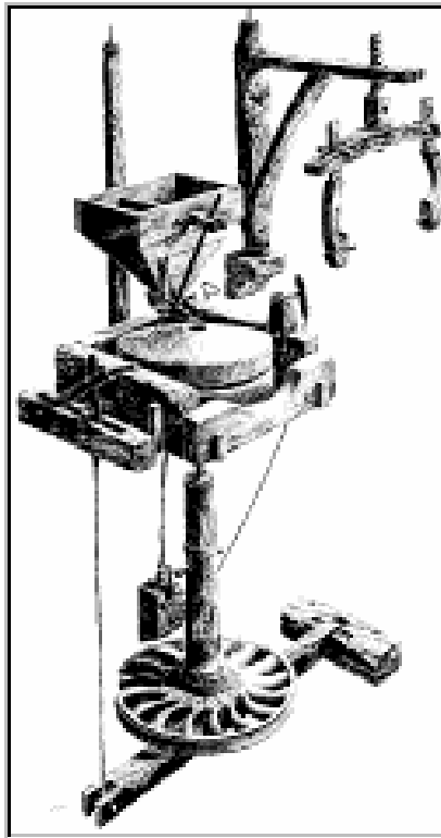
Fig.2. Esquema de un molino de rodezno
