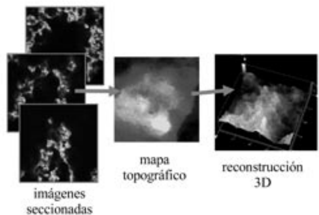
Fig. 2.- Esquema del proceso de reconstrucción topográfica. Se adquieren una serie de imágenes procedentes de la muestra, correspondientes a alturas equiespaciadas del plano focal, y se calcula un mapa topográfico, a partir del cual se obtienen la vista 3D de la superficie y los perfiles que se deseen.
