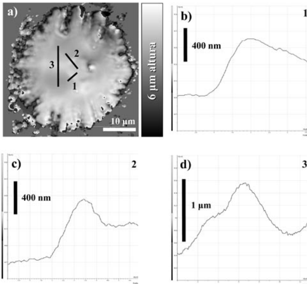
Fig. 8.- Detalle de la fibra 7d. a): Mapa topográfico b), c), d): Perfiles representativos.
