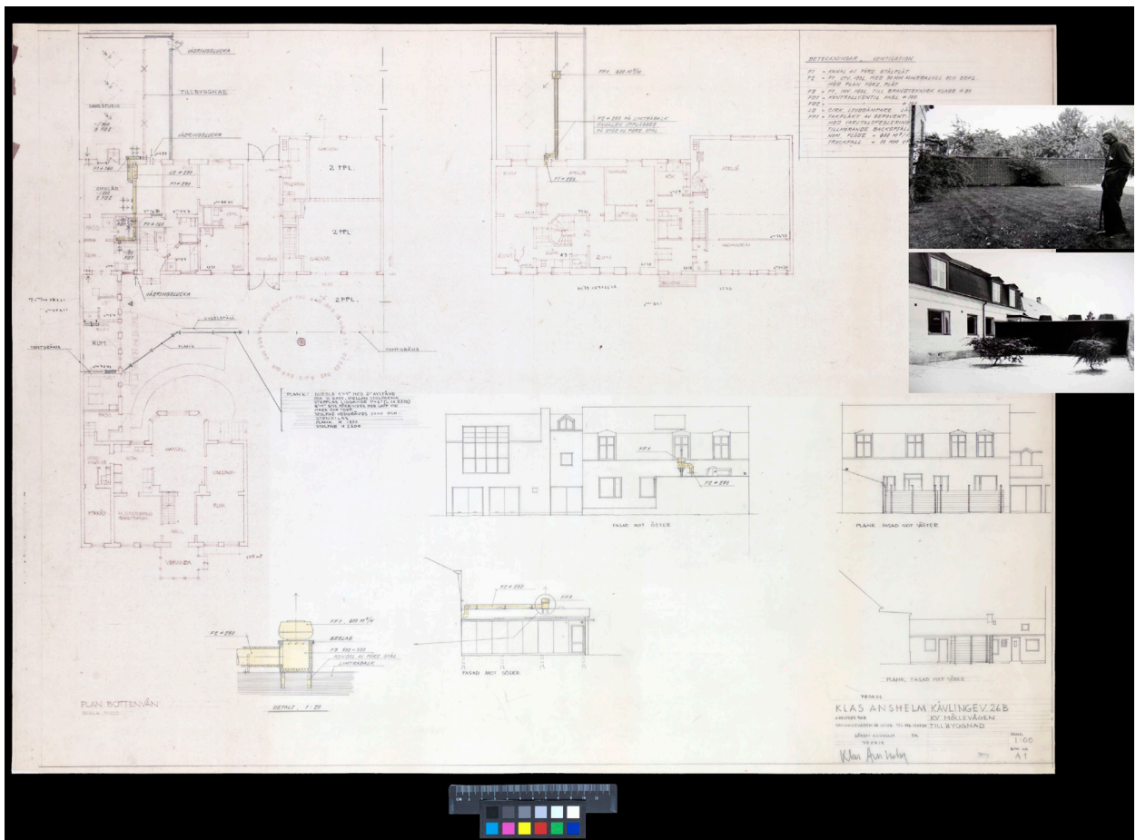
Figura 8. 26 de Kävlingsvägen en Lund, Klass Anshelm, 1970. Planos originales de la casa, entregados en el Ayuntamiento para la construcción de la Black Box. Arriba, el maestro en el jardín trasero; el objeto aún no está construido. Abajo, recién terminada. Fuente: Planimetría e imágenes cedidas por Arkitekturmuseet, Estocolmo.
