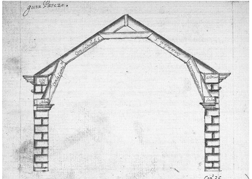
Fig. 3. Armadura de cinco paños.
