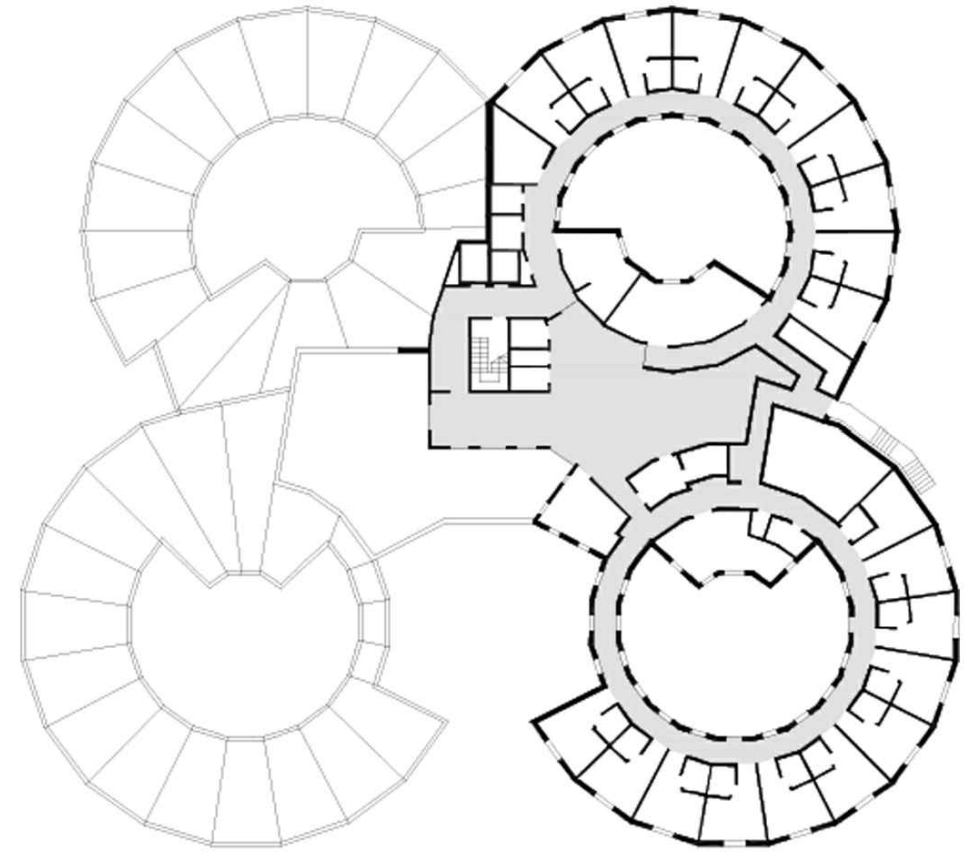
Planta alta
