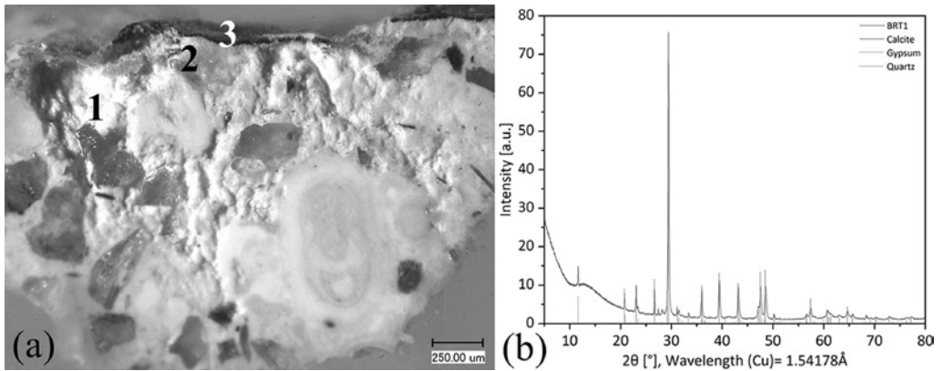
4. (a) Fotografija prečnega prereza vzorca z ometom z OM (1), belo barvno plastjo (ne gre za belež) (2) in črno barvno plastjo (3), (b) XRD graf analize ometa. Sv. Bolfgang, Bad Radkersburg, cerkev sv. Janeza Krstnika
