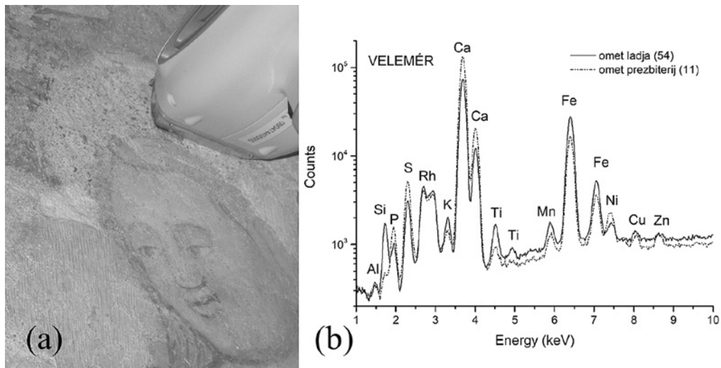
1. (a) In situ XRF analiza ometa, (b) primerjava XRF grafov analize ometa v ladji (54) in prezberiju (11). Marijin nimb, Sv. Ana Samotretja, ladijska slavoločna stena, Velemér, cerkev Marijinega oznanenja
