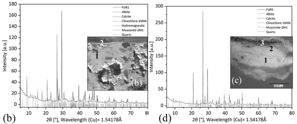
5. (b) XRD graf analize ometa, (b) Fotografija prečnega prereza vzorca z ometom z OM (1) in rdečo barvno plastjo (2). Vera Icon, južno-vzhodni zaključek prezbiterijskega. (c) Fotografija prečnega prereza vzorca z dvema plastema apnenega beleža (1, 2) in vijolično barvno plastjo, (d) XRD graf analize ometa. Apostol v prvem medaljonu, južna stena prezbiterijskega. Furstenfeld, nekdanja samostanska cerkev avguštincev-eremitov
