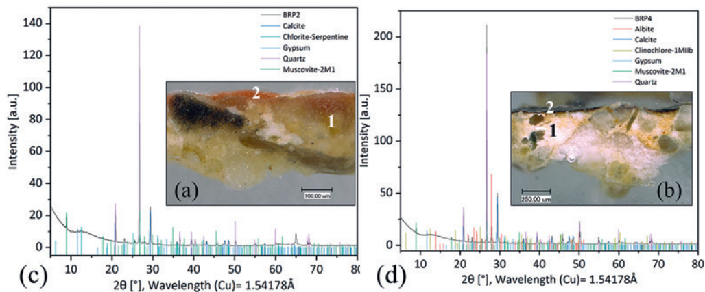
[KRIŽNAR 3] (a) Fotografija prečnega prereza vzorca z ometom z OM (1) in rdečo barvno plastjo (2), (b) XRD graf analize ometa. Priamova smrt, severna stena. (c) Fotografija prečnega prereza vzorca z ometom z OM (1) in črno barvno plastjo (2), (d) XRD graf analize ometa. Mačka z mišjo, južna stena. Bad Radkersburg. Pistorjeva hiša
