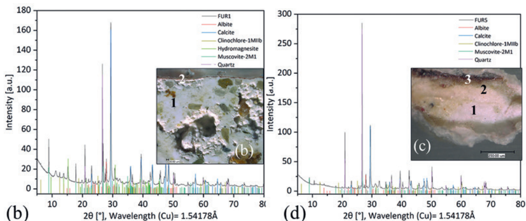
[KRIŽNAR 5] (b) XRD graf analize ometa, (b) Fotografija prečnega prereza vzorca z ometom z OM (1) in rdečo barvno plastjo (2). Vera Icon, južno-vzhodni zaključek prezbiterja. (c) Fotografija prečnega prereza vzorca z dvema plastema apnenega beleža (1, 2) in vijolično barvno plastjo, (d) XRD graf analize ometa. Apostol v prvem medaljonu, južna stena prezbiterja. Furstenfeld, nekdanja samostanska cerkev avguštincev-eremitov
