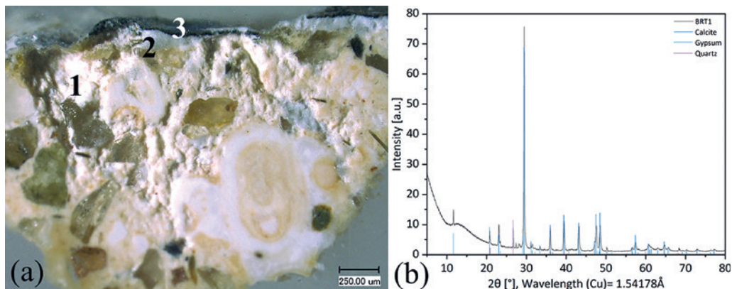
[KRIŽNAR 4] (a) Fotografija prečnega prereza vzorca z ometom z OM (1), belo barvno plastjo (ne gre za belež) (2) in črno barvno plastjo (3), (b) XRD graf analize ometa. Sv. Bolfgang, Bad Radkersburg, cerkev sv. Janeza Krstnika
