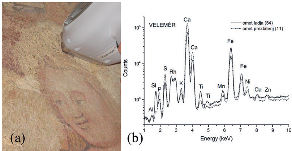
[KRIŽNAR 1] (a) In situ XRF analiza ometa, (b) primerjava XRF grafov analize ometa v ladji (54) in prezbiteriju (11). Marijin nimb, Sv. Ana Samotretja, ladijska slavoločna stena, Velemér, cerkev Marijinega oznanjenja
