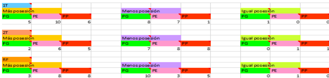
Figura 25. Relación posesión de balón – resultado del Athletic Club.
