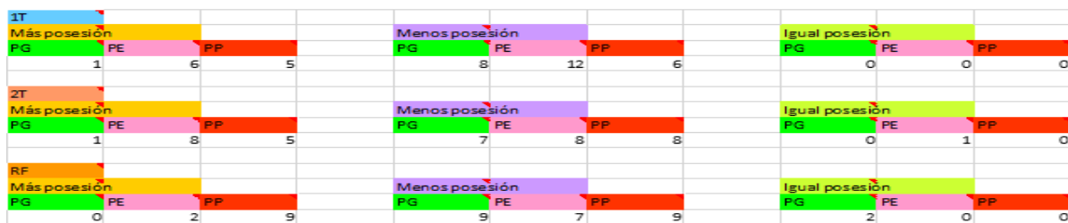
Figura 31. Relación posesión de balón – resultado del Eibar.
