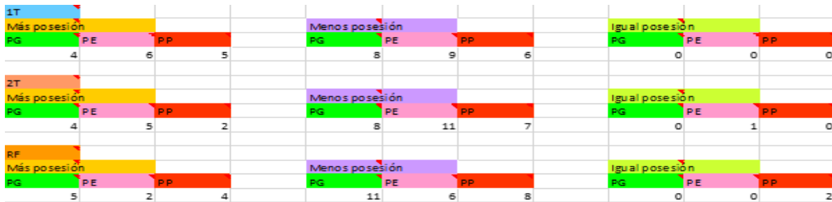
Figura 17. Relación posesión de balón – resultado del Granada.
