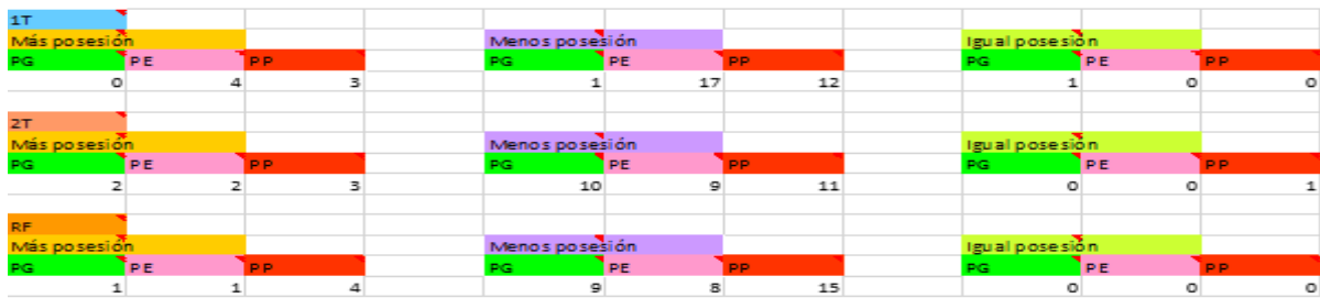
Figura 35. Relación posesión de balón – resultado del Alavés.
