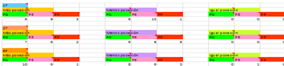
Figura 9. Relación posesión de balón – resultado del Atlético de Madrid.
