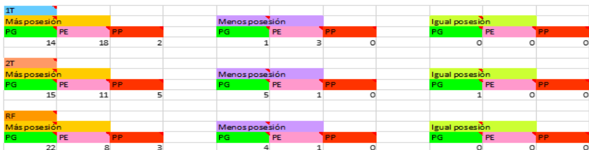
Figura 5. Relación posesión de balón – resultado del Real Madrid
