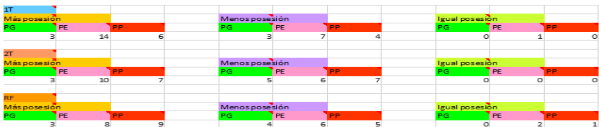
Figura 37. Relación posesión de balón – resultado del Celta de Vigo.
