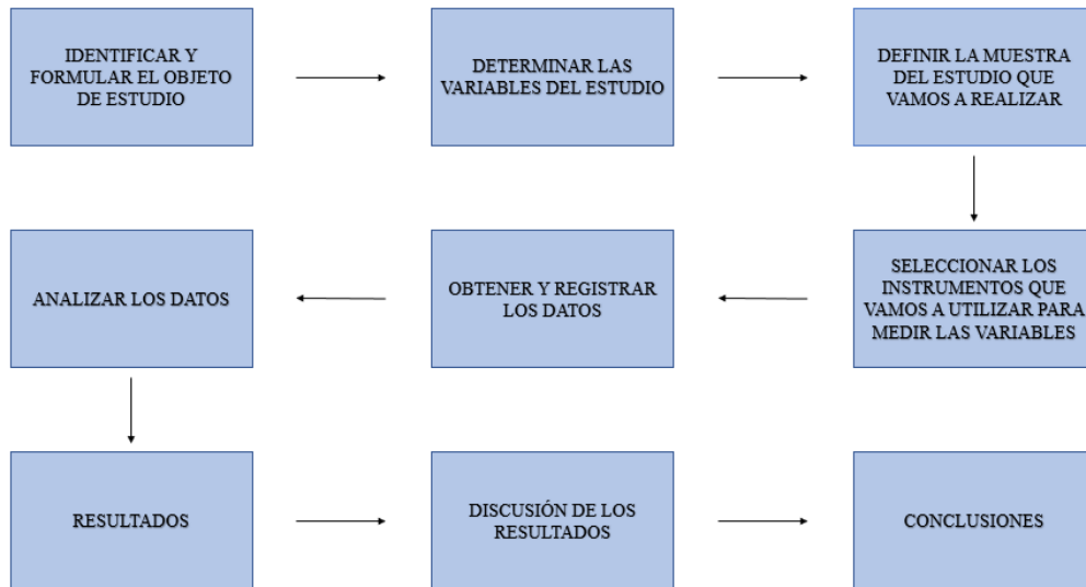
Figura 1. Fases del diseño de investigación
