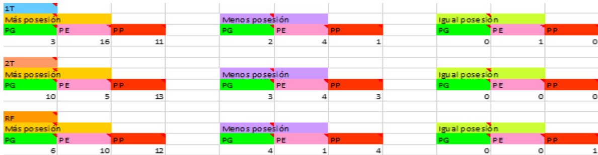
Figura 33. Relación posesión de balón – resultado del Real Betis.
