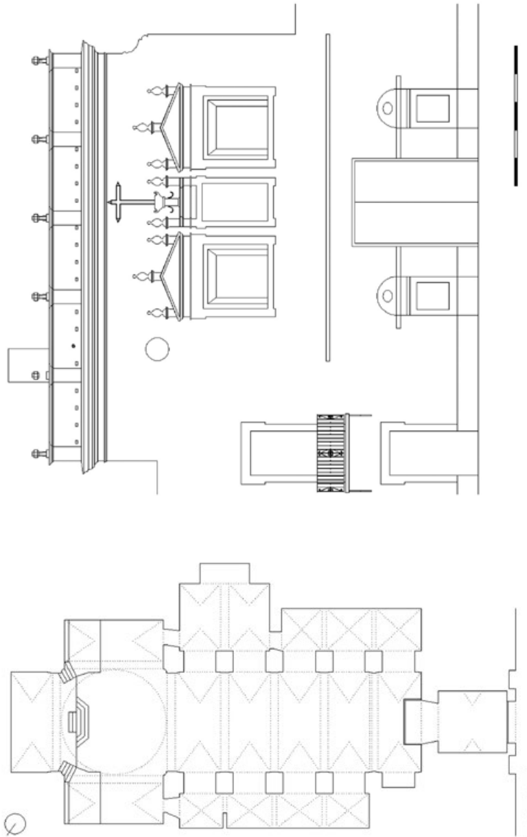
Figuras 7 y 8. Planta y alzado de la fachada de los pies de la iglesia del extinto convento de San Diego, levantados por la arquitecta D a Silvia Macarena Montalbán Arévalo.
