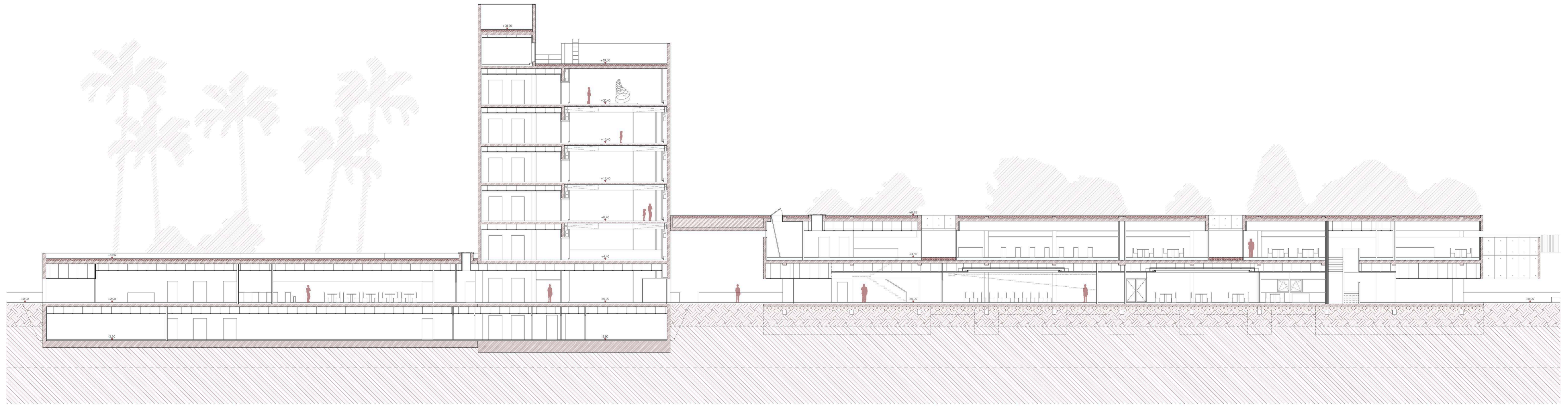
SECCIÓN B-B'
