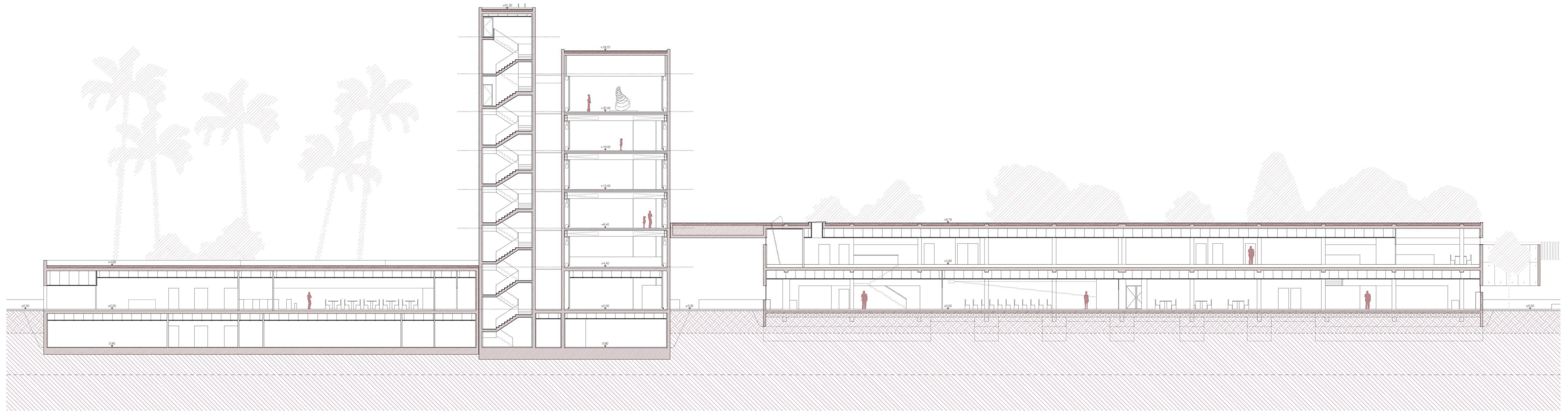
SECCIÓN C-C'
