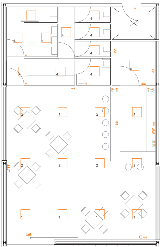
PLANTA RESTAURANTE 1. ESCALA 1:50
