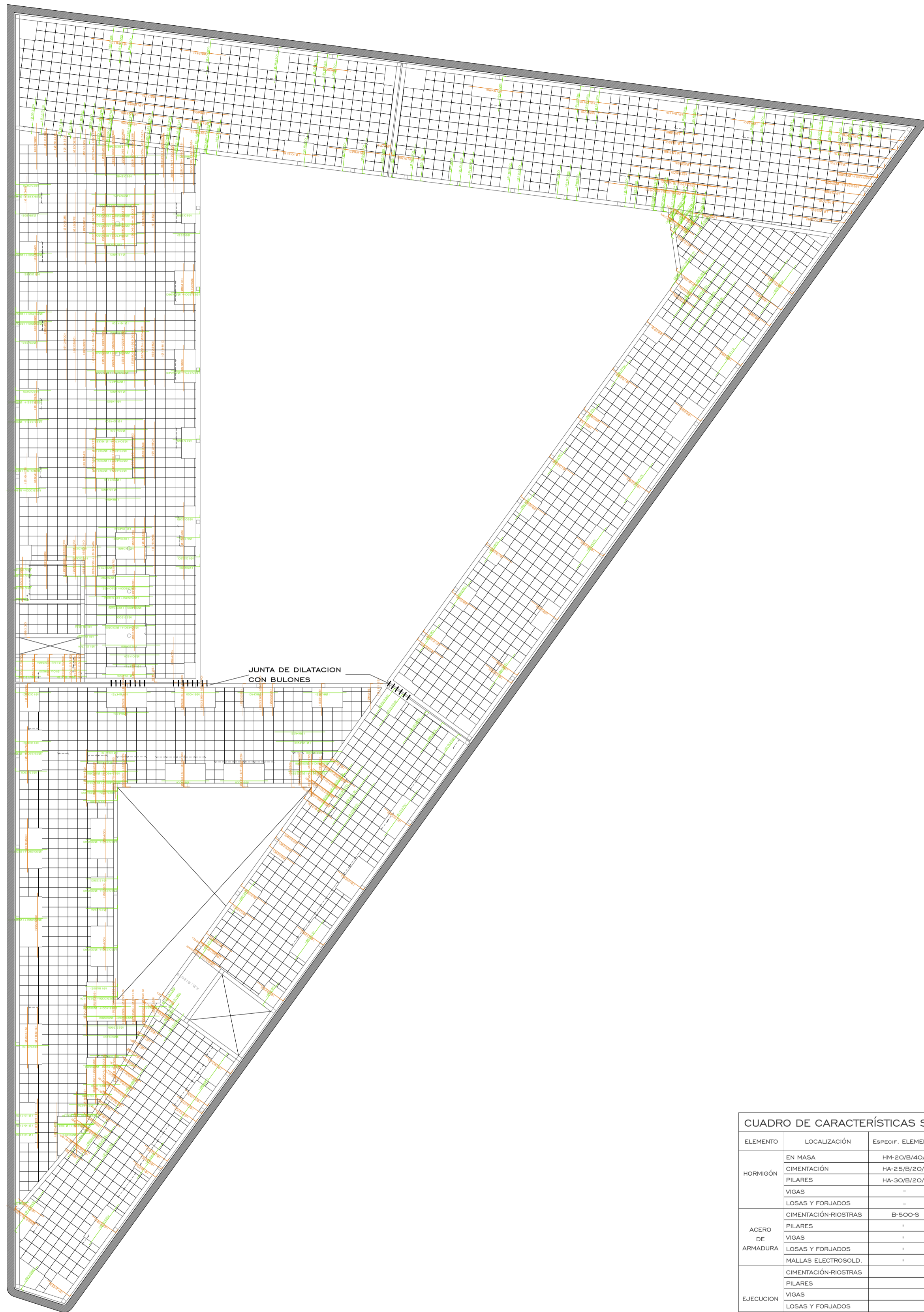
FORJADO REFUERZO SUPERIOR COTA +9,56M E: 1/250
