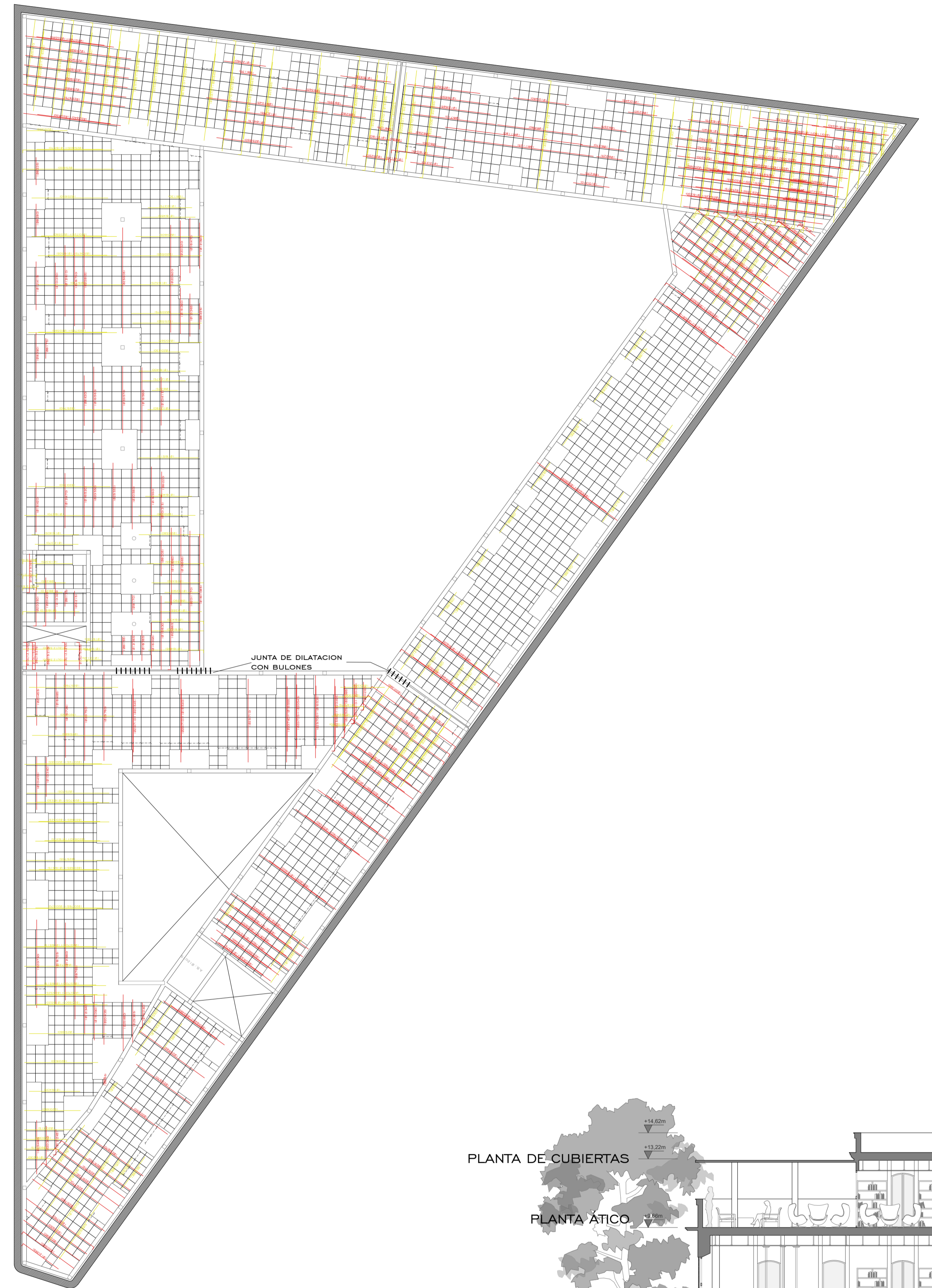
FORJADO REFUERZO INFERIOR COTA +9,56M E: 1/250
