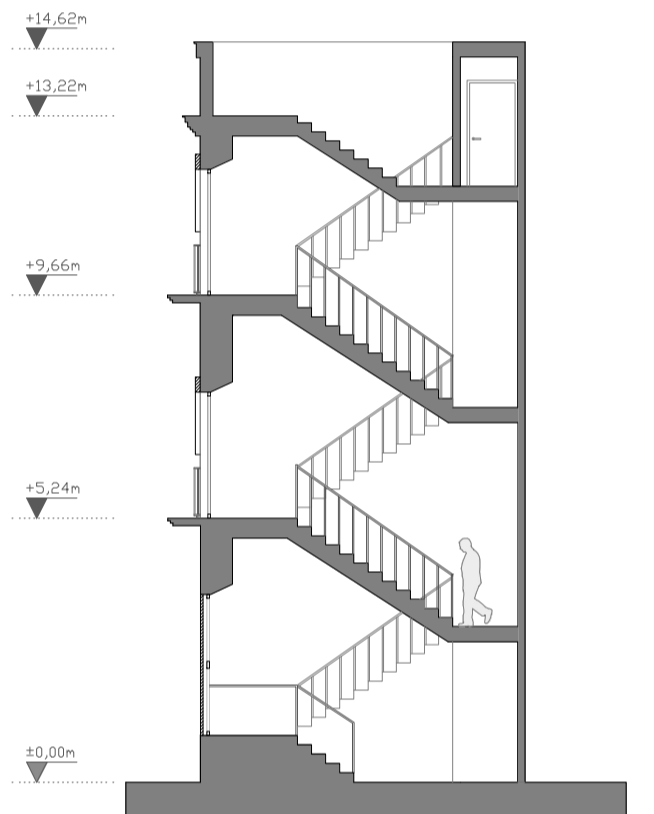
SECCIÓN ESCALERAS
