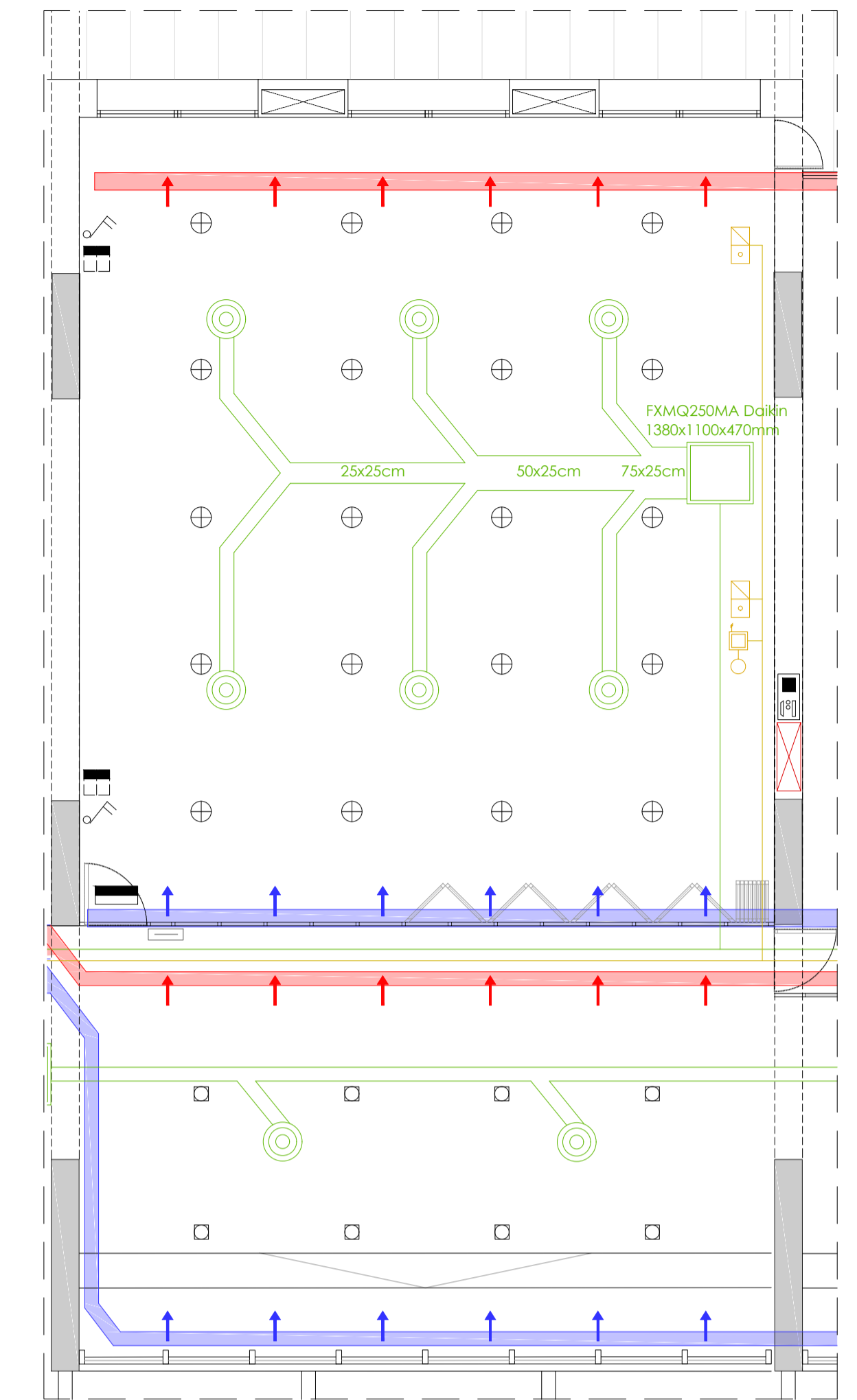
ZOOM DE FALSO TECHO DE AULA Y ESPACIO DE GRADERÍO
