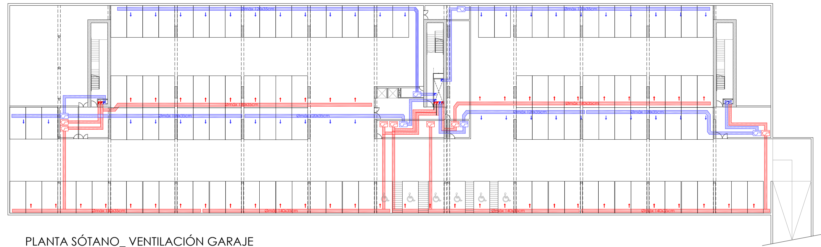
PLANTA SÓTANO_ VENTILACIÓN GARAJE
