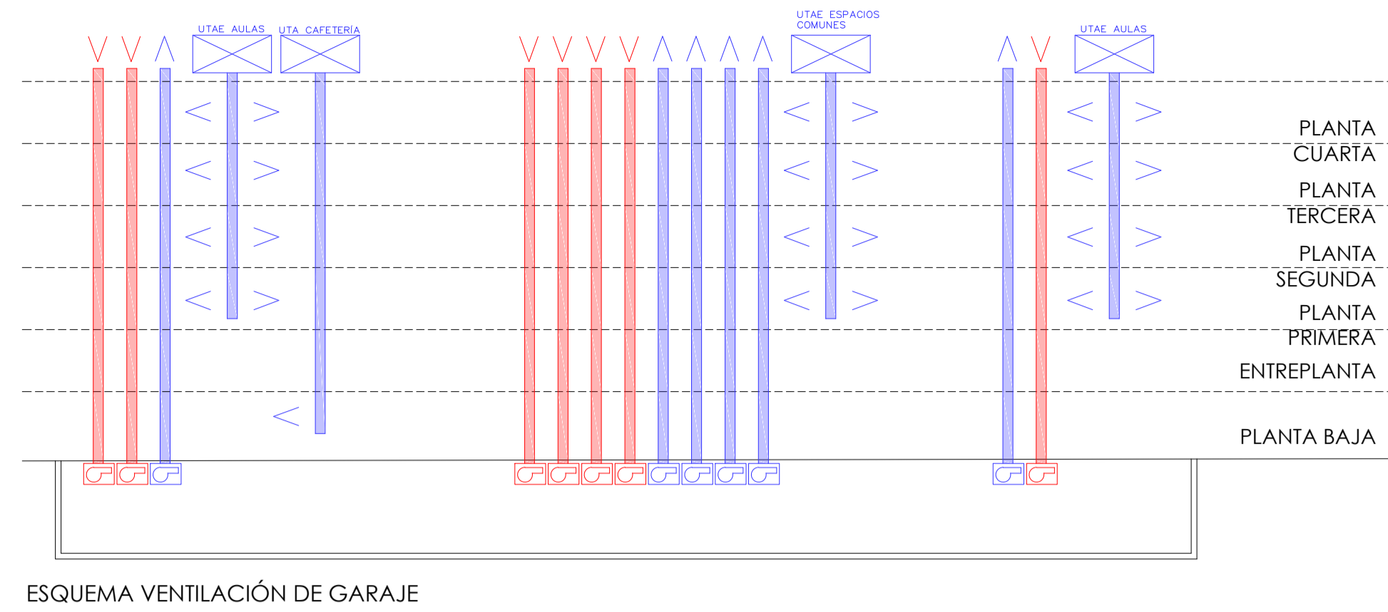
ESQUEMA VENTILACIÓN DE GARAJE
