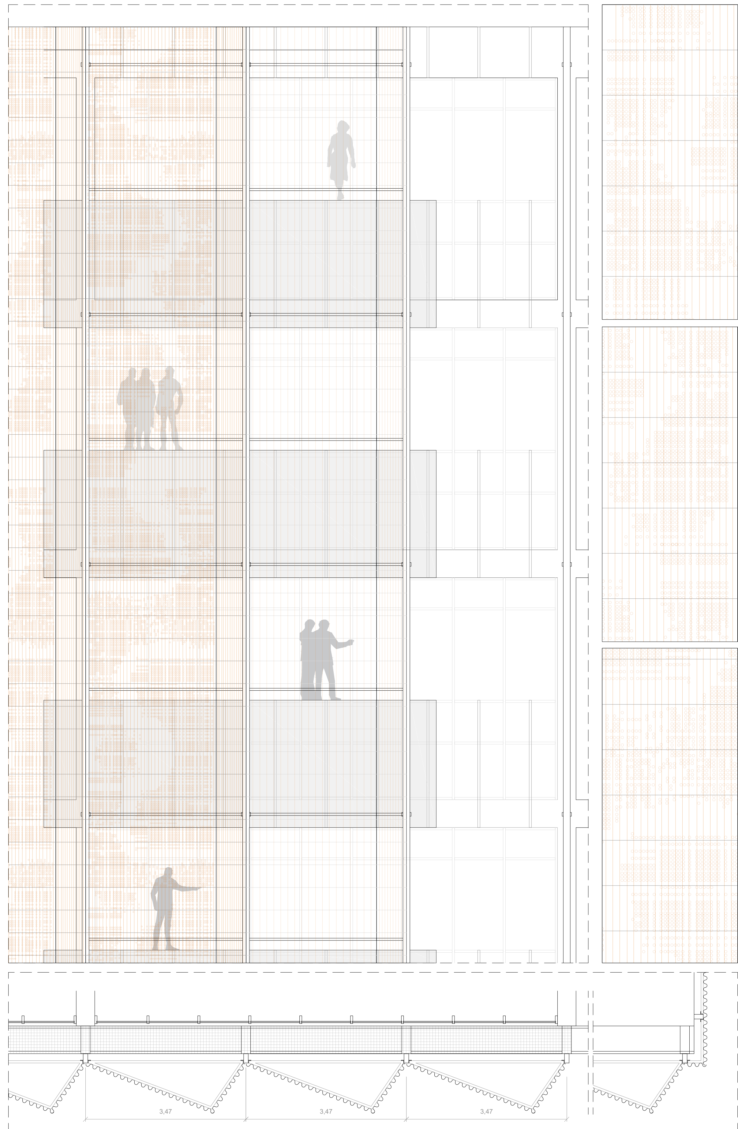
ALZADO Y PLANTA DEL DESPIECE DE LA FACHADA OESTE. FACHADA DE COBRE. DETALLES DE LAS PERFORACIONES DE LA FACHADA DE COBRE (ESCALA 1:25)
