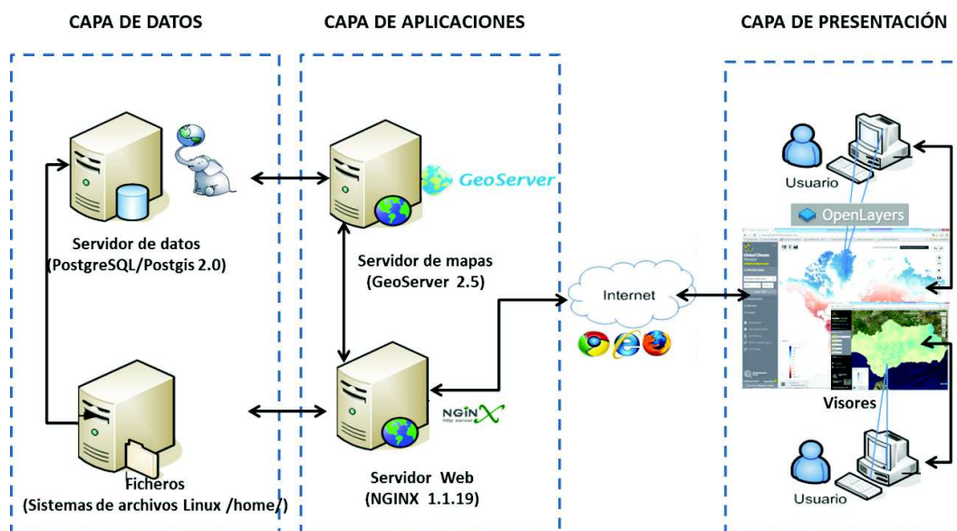
Fig. 1. Arquitectura del sistema Cambia. Fuente: Elaboración propia.
