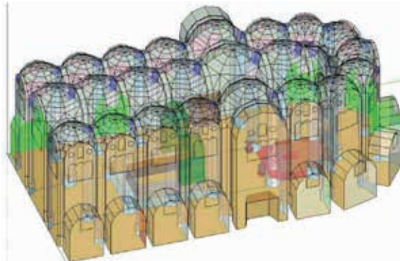
FIGURA 8: Fuente: elaboración propia; Nota pie de figura: Modelo 3D de la catedral de Málaga implementado para la simulación.
