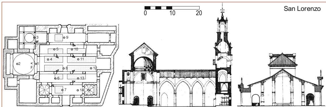
Figura 13. Planta, con la ubicación de los receptores (O), de la fuente (F) y de los altavoces del sistema electroacústico existente (D), y secciones longitudinal y transversal de la Iglesia de San Lorenzo.
