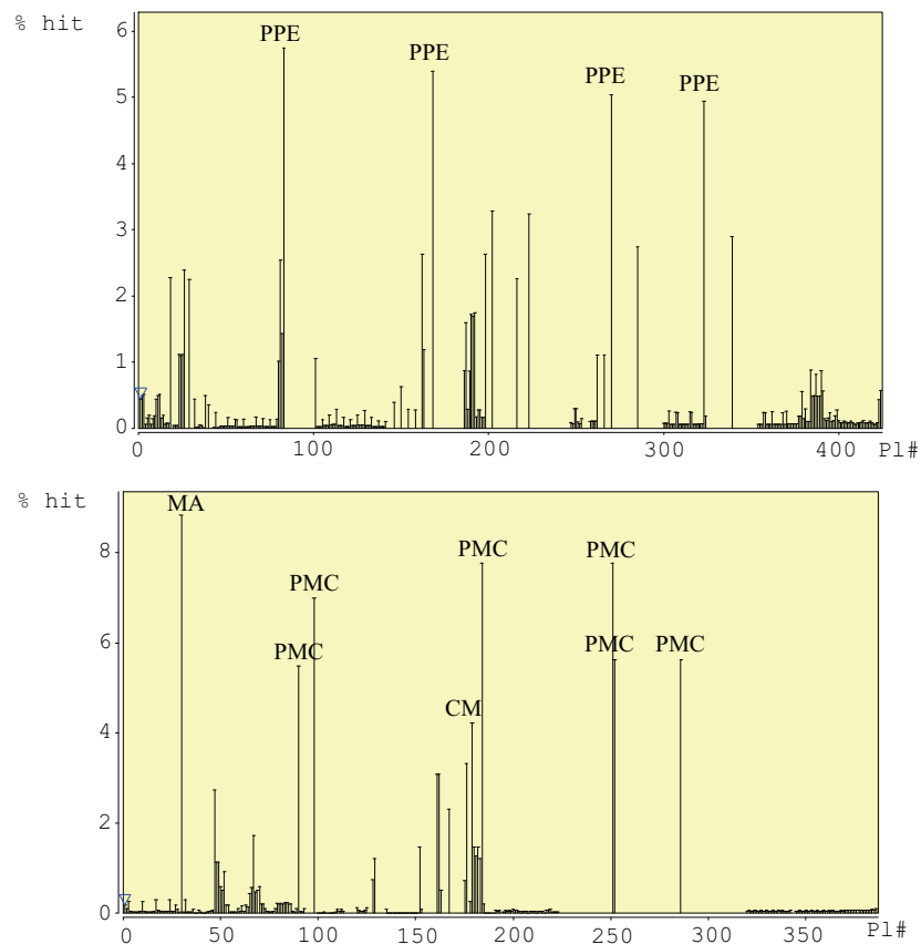
Figura 6. Histogramas de reflexiones producidas en las superficies (identificadas por el número asignado en el modelo): para la iglesia de San Pedro (arriba) y la de San Marcos (abajo). Los materiales de las superficies más significativas (con un porcentaje superior al 4%) se identifican en cada caso con el acrónimo asignado en la Tabla 1.
