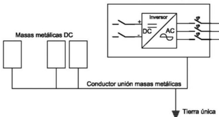
Ilustración 2.7 Esquema puesta a tierra para instalación tipo IT.
