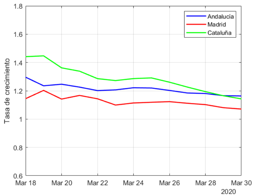
Figura 3. Tasa de crecimiento estimada para diferentes comunidades
