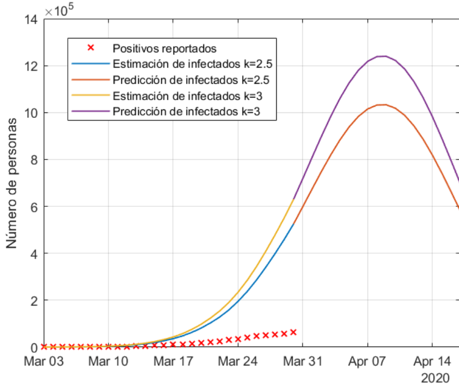
Figura 6. Estimación y predicción de infectados para diferentes valores de k
