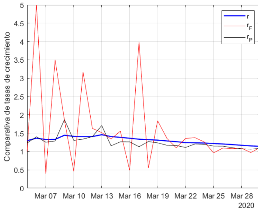
Figura 1. Comparación de las tasas de crecimiento obtenidas con datos publicados y mediante filtro de Kalman para el territorio español
