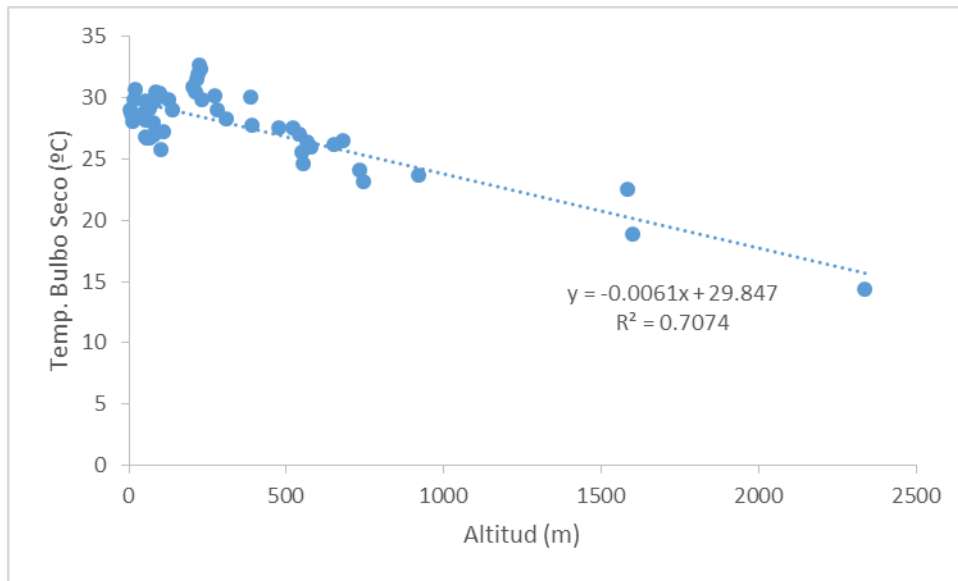
Figura 15 Correlación entre DBT y la Altura. Fuente Propia.
