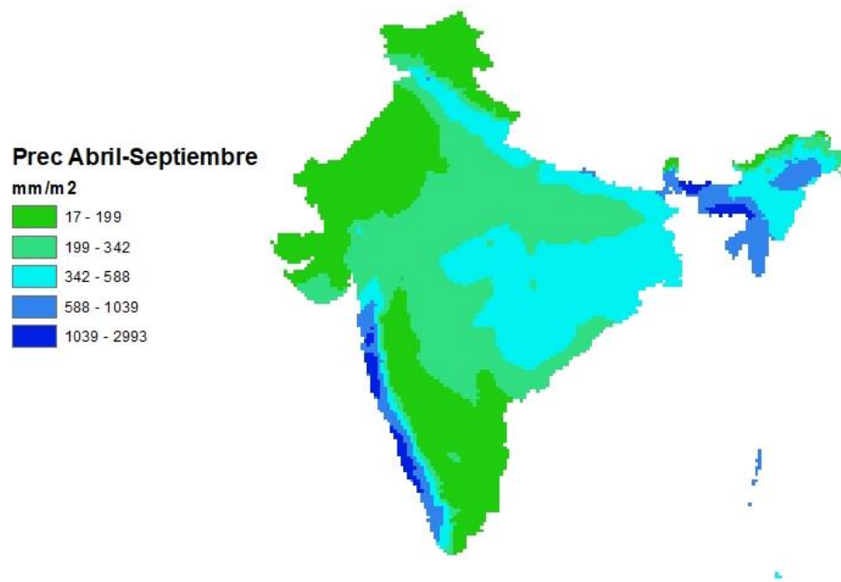
Figura 32 Mapa de precipitaciones acumuladas entre los meses de Abril a Septiembre. Fuente Propia.
