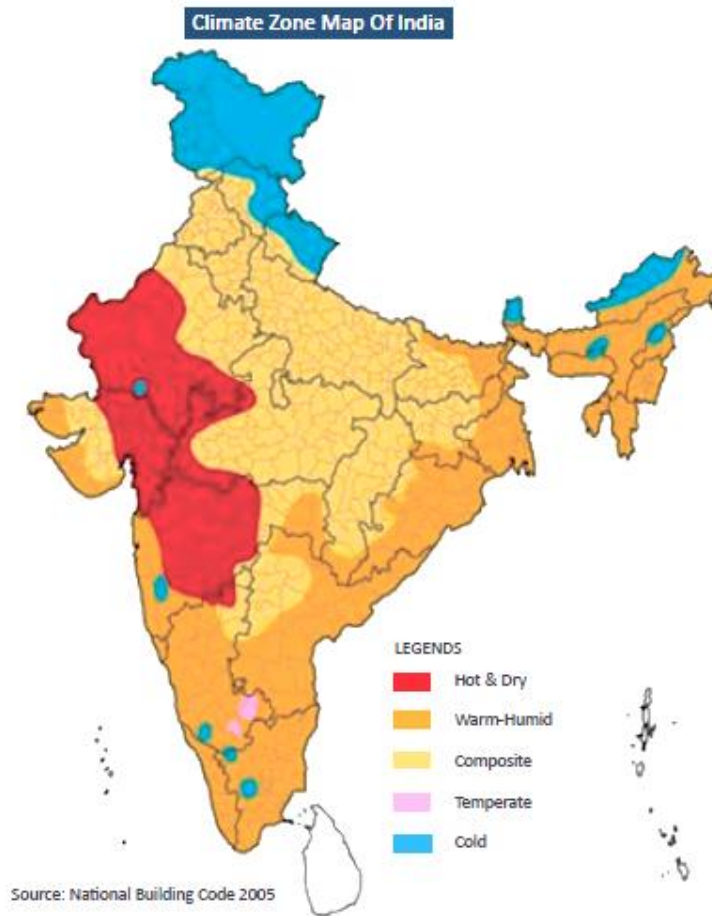
Figura 11 Mapa de Zona Climática de India. Fuente National Building Code 2005.
