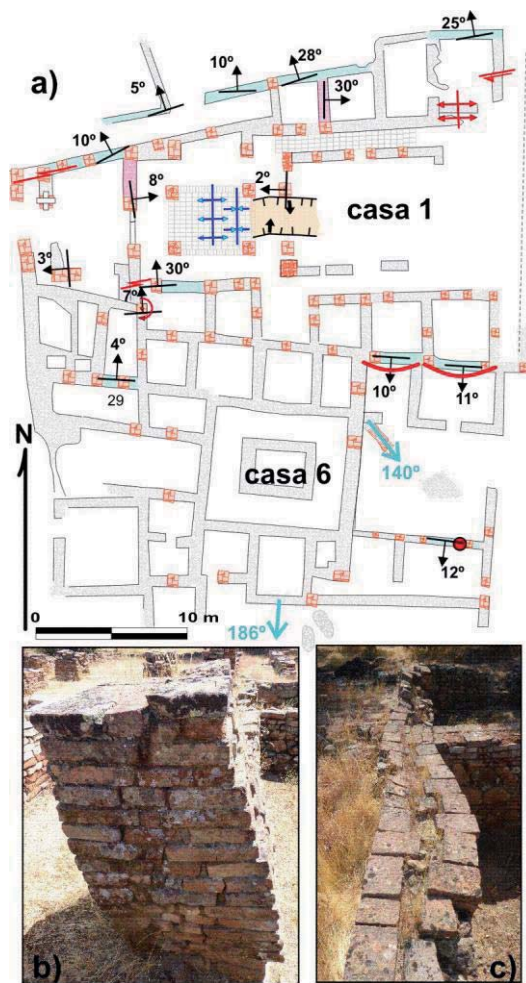
FIGURA 5. a) Cartografía de los EAEs en las casas 1 y 6 (Giner-Robles et al., inédito). Las principales estructuras inventariadas en esta casa son basculamientos y colapsos de muros y caídas orientadas (pilares de ladrillo). b) Basculamiento de uno de los pilares de ladrillo de la casa 1. c) Muro plegado y desplazado en el límite de la casa 1 con la casa 6 (ver Fig.1).
