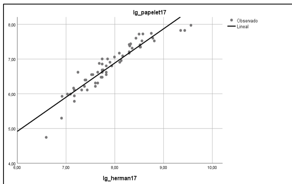
Figura 3.12. Representación del modelo de elasticidad constante para el año 2017. Fuente: Elaboración propia.
