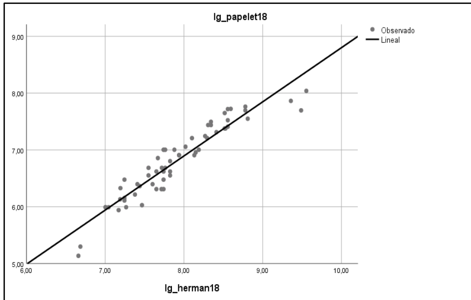
Figura 3.15. Representación del modelo de elasticidad constante para el año 2018. Fuente: Elaboración propia.
