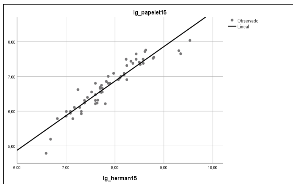
Figura 3.6. Representación del modelo de elasticidad constante para el año 2015. Fuente: Elaboración propia.
