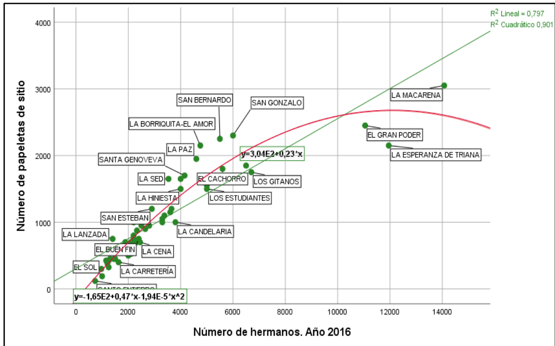
Figura 3.8. Representación de los dos ajustes para el año 2016.
