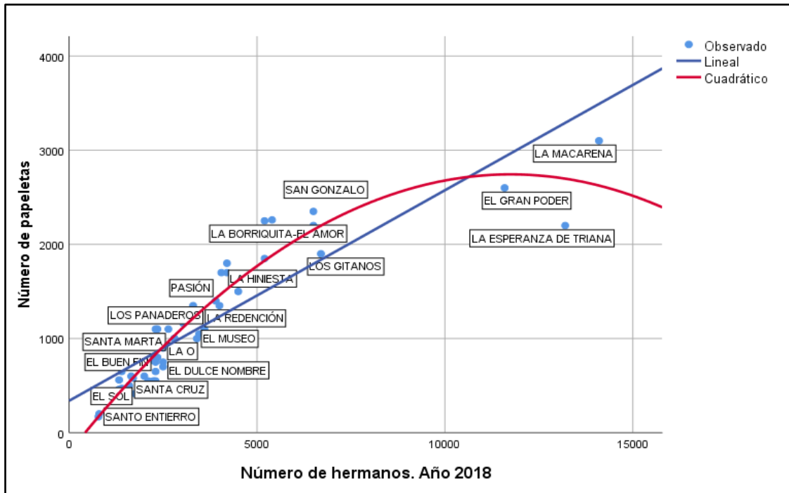
Figura 3.14. Representación de los dos ajustes para el año 2018.
