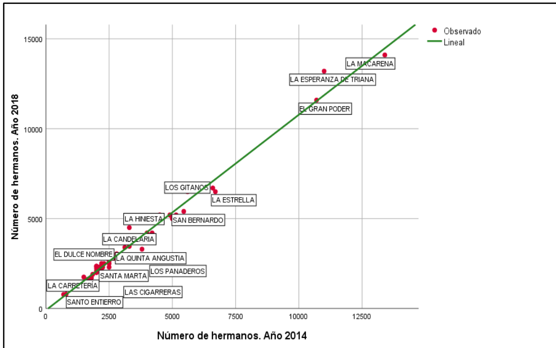
Figura 3.16. Representación del ajuste lineal para todo el periodo de estudio. Fuente: Elaboración propia.
