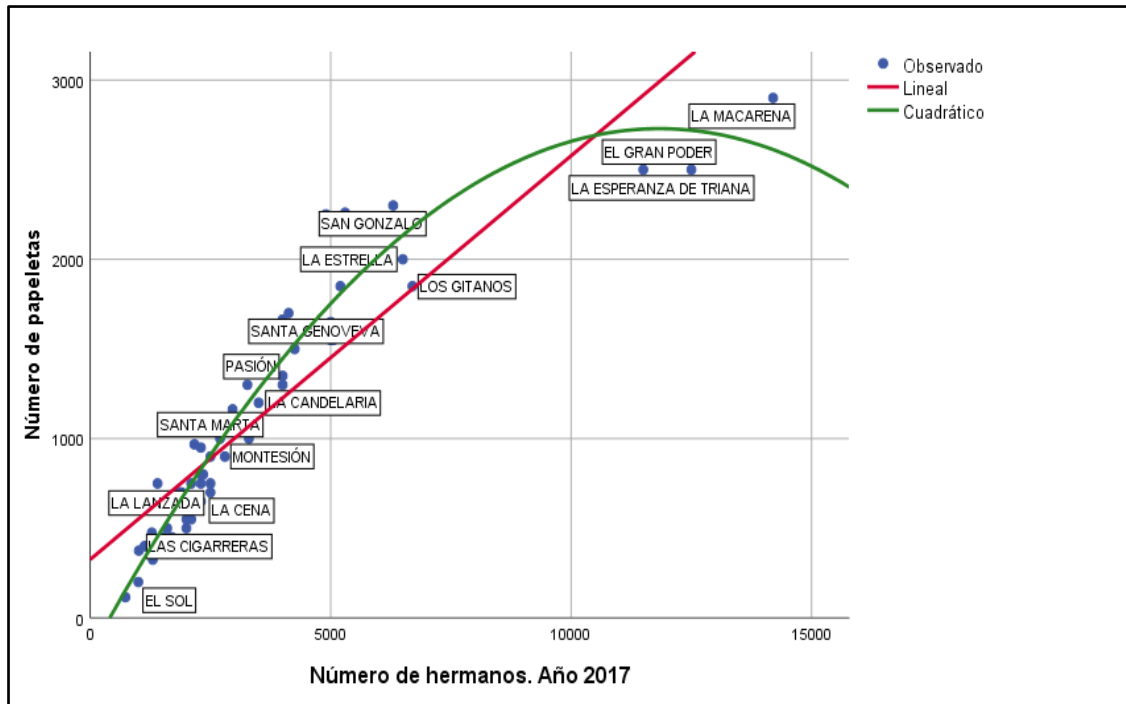
Figura 3.11. Representación de los dos ajustes para el año 2017.
