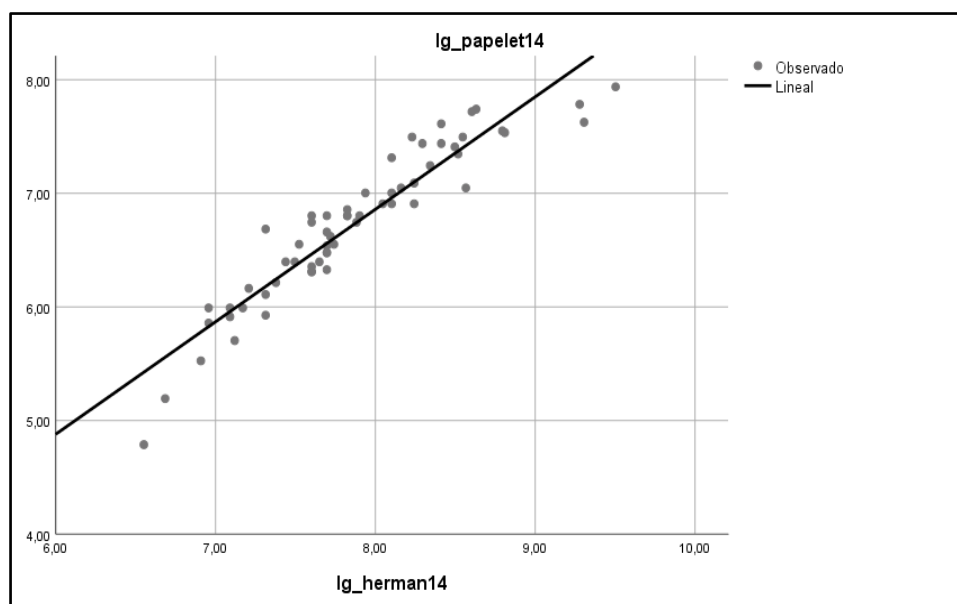
Figura 3.3. Representación del modelo de elasticidad constante para el año 2014. Fuente: Elaboración propia.
