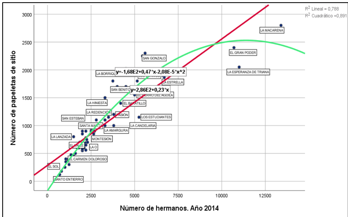
Figura 3.2. Representación de los dos ajustes para el año 2014.
