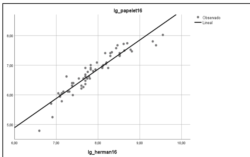
Figura 3.9. Representación del modelo de elasticidad constante para el año 2016. Fuente: Elaboración propia.
