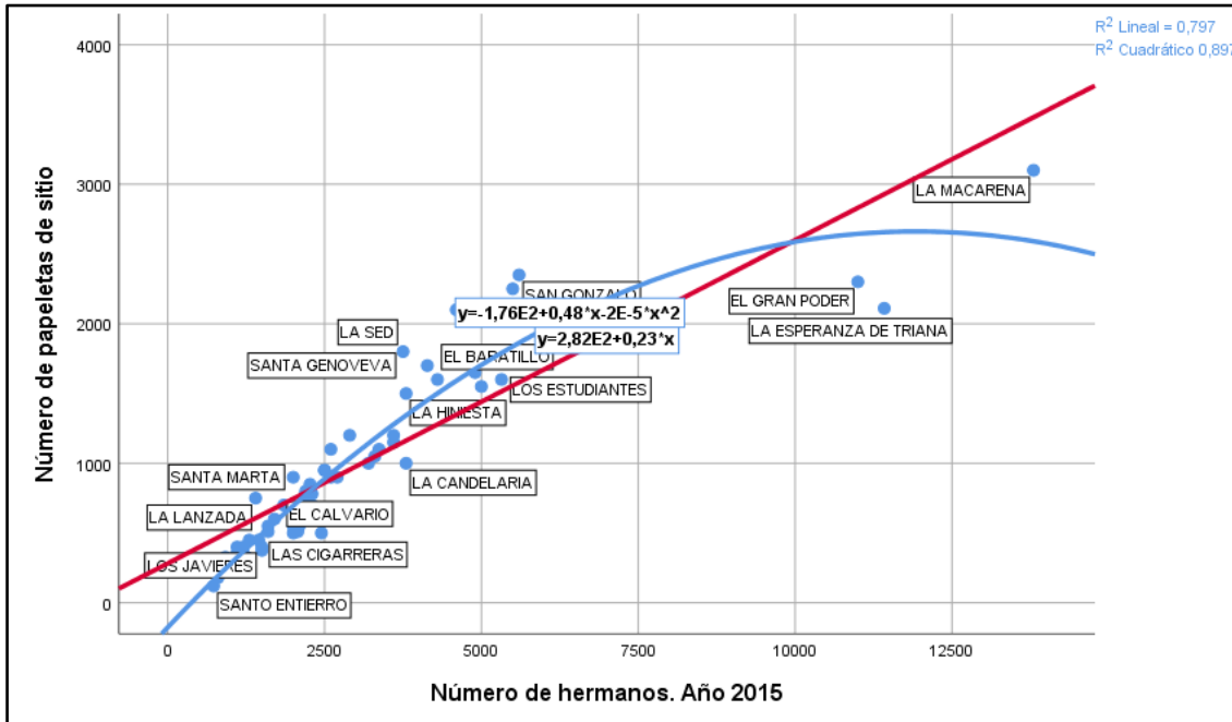
Figura 3.5. Representación de los dos ajustes para el año 2015.
