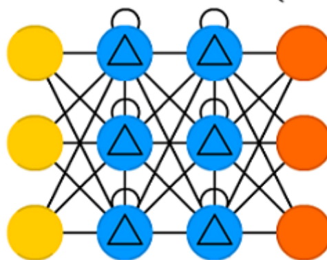
Figura 4.5: GRU
