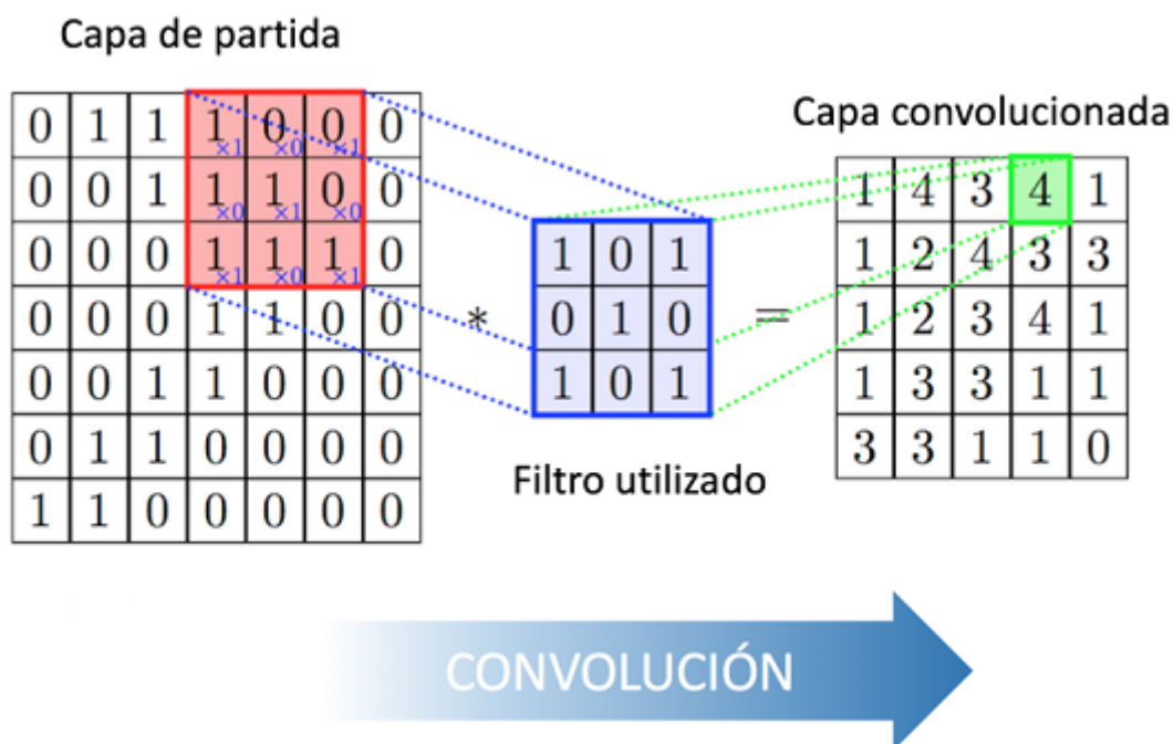
Figura 4.7: Convolución CNN
