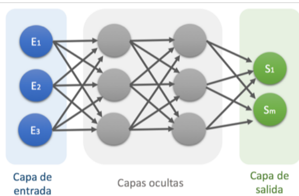
Figura 2.7: Perceptrón Múltiple
