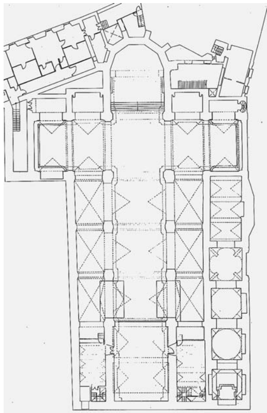
Figura 4 Planta alta del actual del templo. Leonardo de Figuroa 1690-1703.
