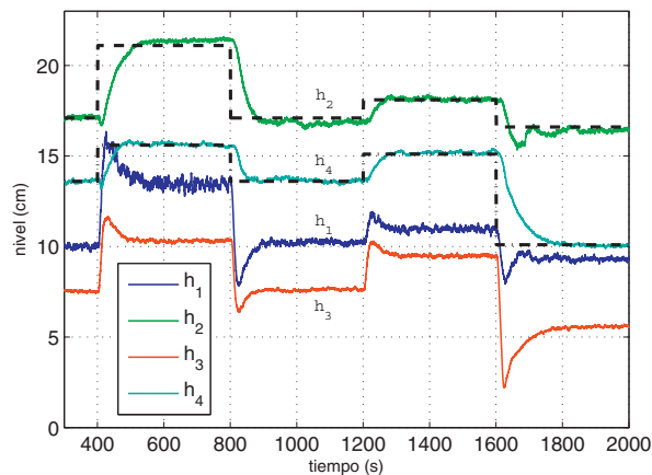
Figura 3: Seguimiento de referencias con muestreo periódico. Las referencias están con líneas de trazos.
