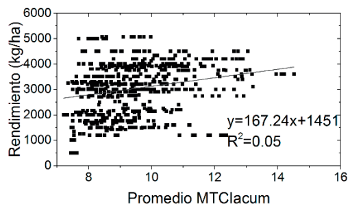
Figura 6. Diagramas de dispersión entre el rendimiento procedente de ESYRCE y el promedio del índice MTCIacum, para cada recinto SIGPAC de los segmentos territoriales muestreados por ESYRCE.
