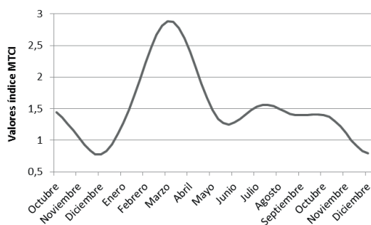
Figura 2. Perfil del índice MTCI en una parcela de trigo de Utrera (Sevilla) en 2006-2007.
