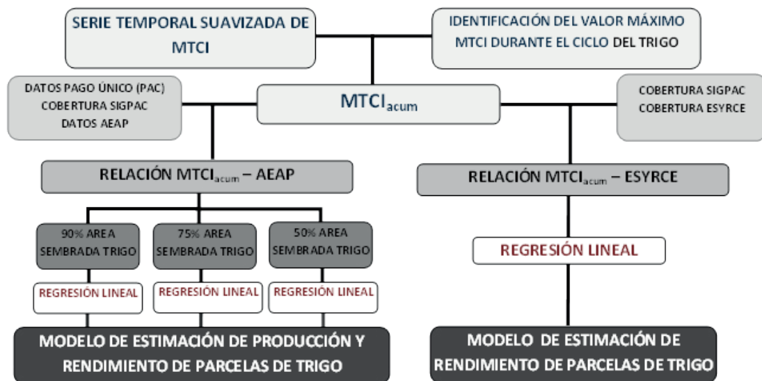
Figura 1. Metodología para la obtención de modelos de estimación de cosecha para el periodo comprendido entre 2006 y 2011. Donde: MTCI_{acum} es el sumatorio de MTCI de los 30 días posteriores al máximo valor MTCI, PAC es Política agraria común, SIGPAC es el sistema de información geográfica de parcelas agrícolas, AEAP es el Anuario de estadísticas agrarias y pesqueras de Andalucía, ESYRCE es la Encuesta de superficie y rendimiento de los cultivos.
