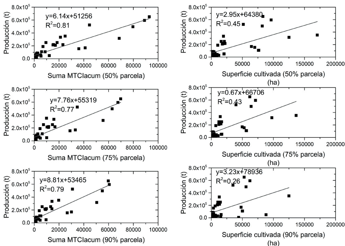
Figura 4. Diagramas de dispersión entre la producción procedente del AEAP y el sumatorio provincial del índice MTCIacum (izquierda) o la superficie total cultivada obtenida del cruce de información entre el SIGPAC-PAC (derecha).
