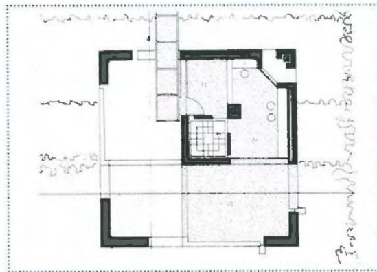
Fig. 13.- Mario BOTTA, Vivienda unifamiliar en Riva San Vitale, Suiza (1972-73)
