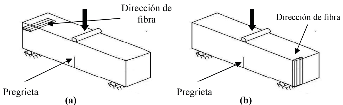
Fig. 1. Probetas con distintas direcciones de fibra con respecto al crecimiento de grieta: (a) crecimiento perpendicular a la dirección de fibra, (b) crecimiento paralelo a la dirección de fibra
