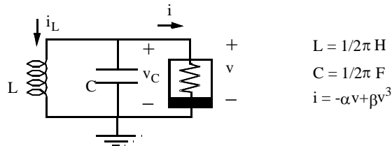
Figura 1. Circuito RLC no lineal.
