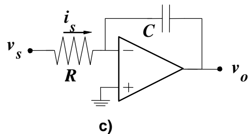
Figura 2. a) Esquema del sumador/escalador y casos contemplados. b) Esquema del diferenciador. c) Esquema del integrador.
