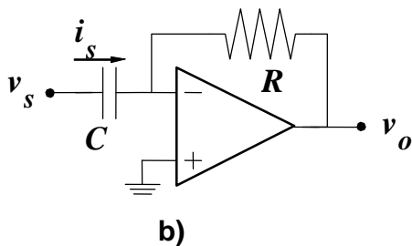
Figura 2. a) Esquema del sumador/escalador y casos contemplados. b) Esquema del diferenciador. c) Esquema del integrador.
