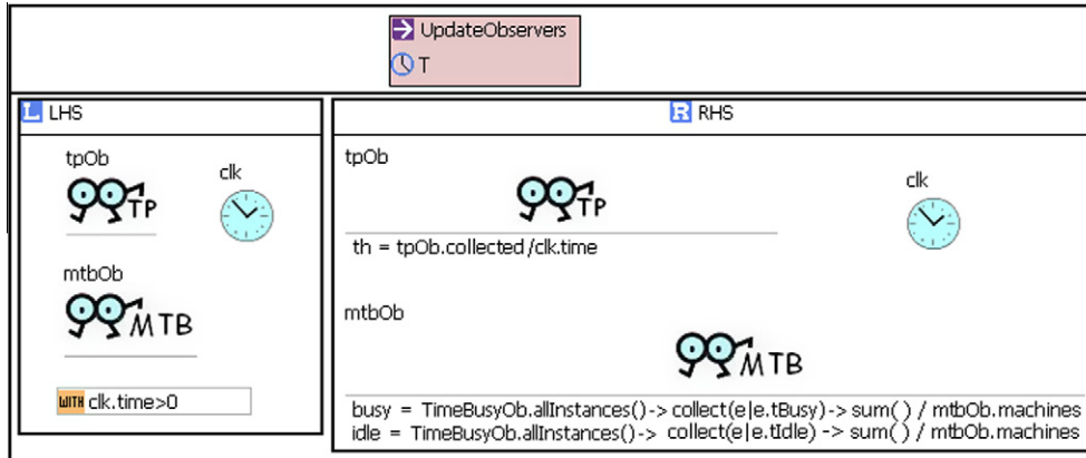
Fig. 12. UpdateObservers rule.
