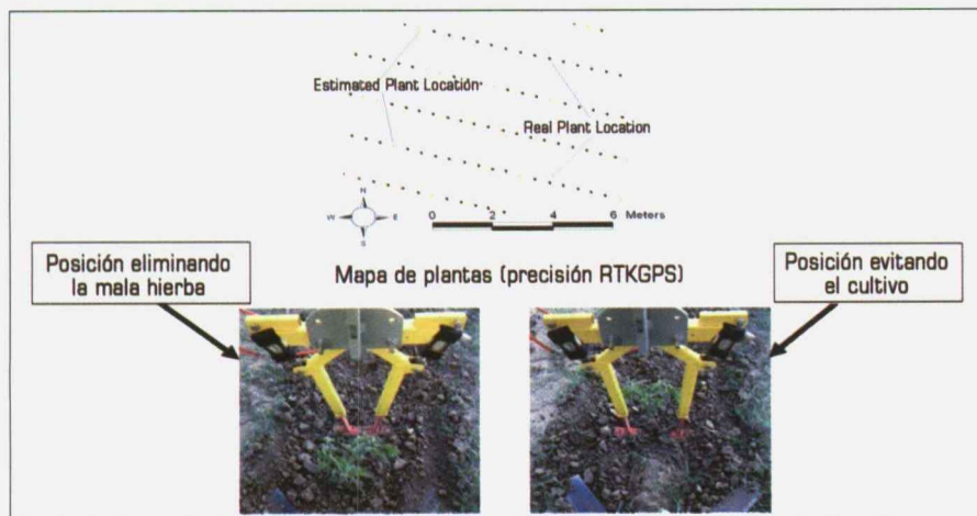
Escarda mecánica en la línea del cultivo con cuchilla neumática utilizando mapa de plantas de alta precisión (Sun et al. , 2010; Slaughter et al. , 2010).
