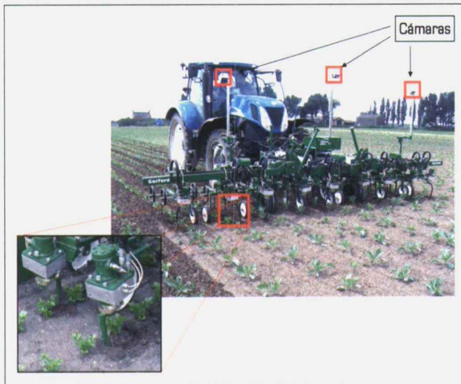
Equipo Robocrop InRow de la compañía Garford (www.garford.com).
