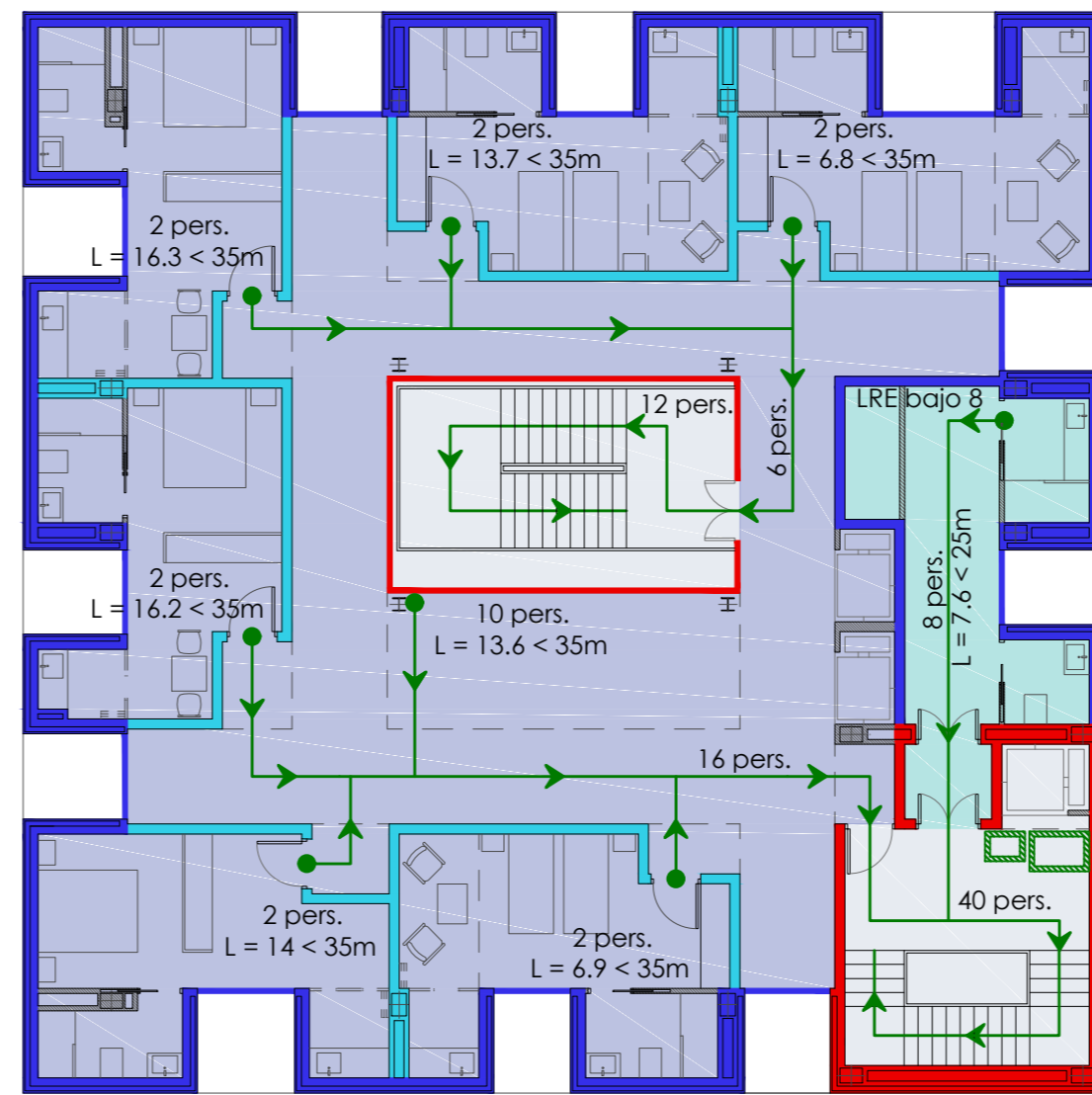
Planta Quinta
