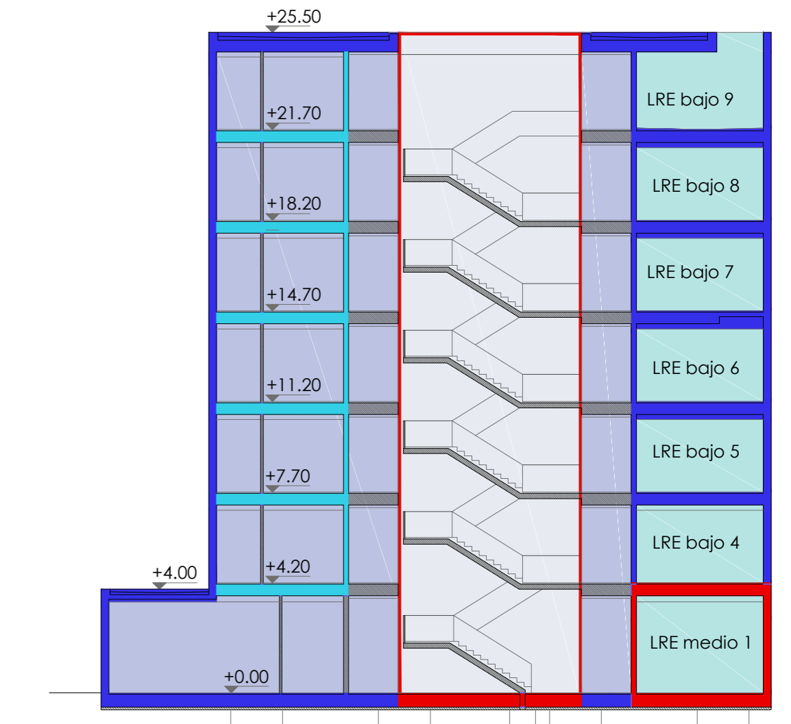
Sección escala 1:200
