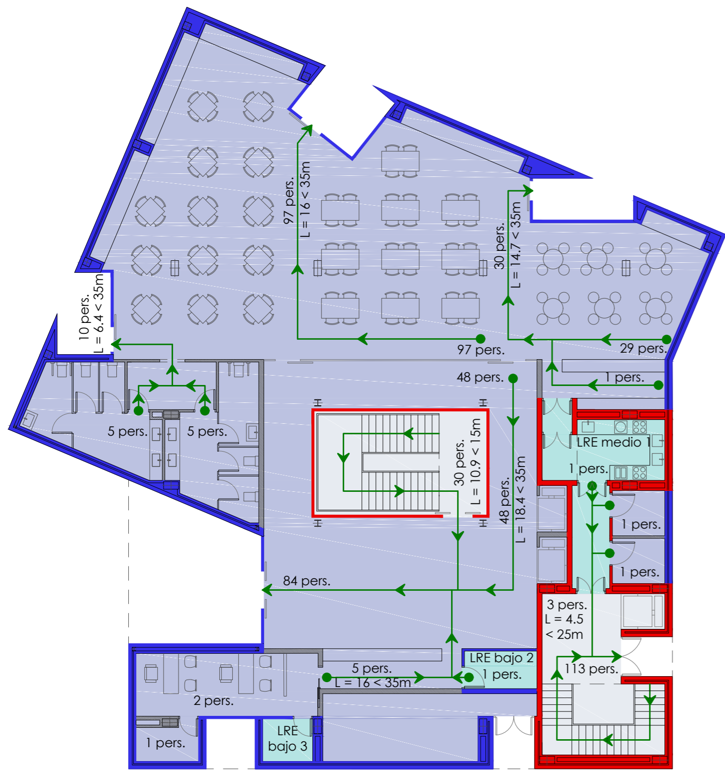
Planta Baja
