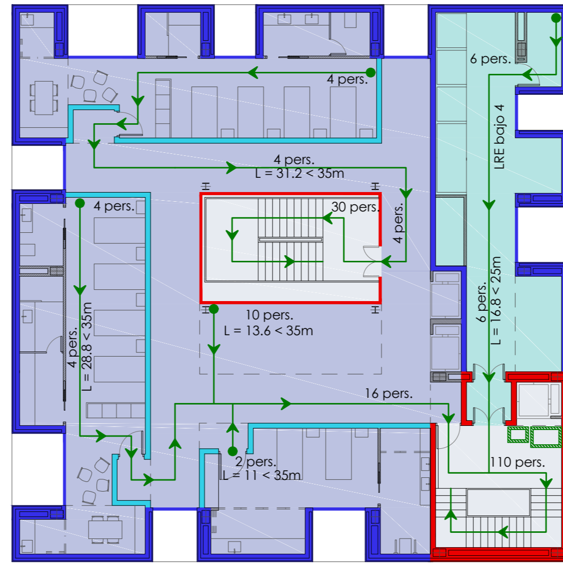
Planta Primera
