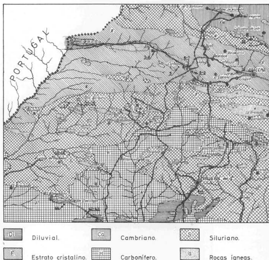
FIG. 1.—Croquis del mapa geológico de la zona en que se encuentran los materiales que se estudian.
