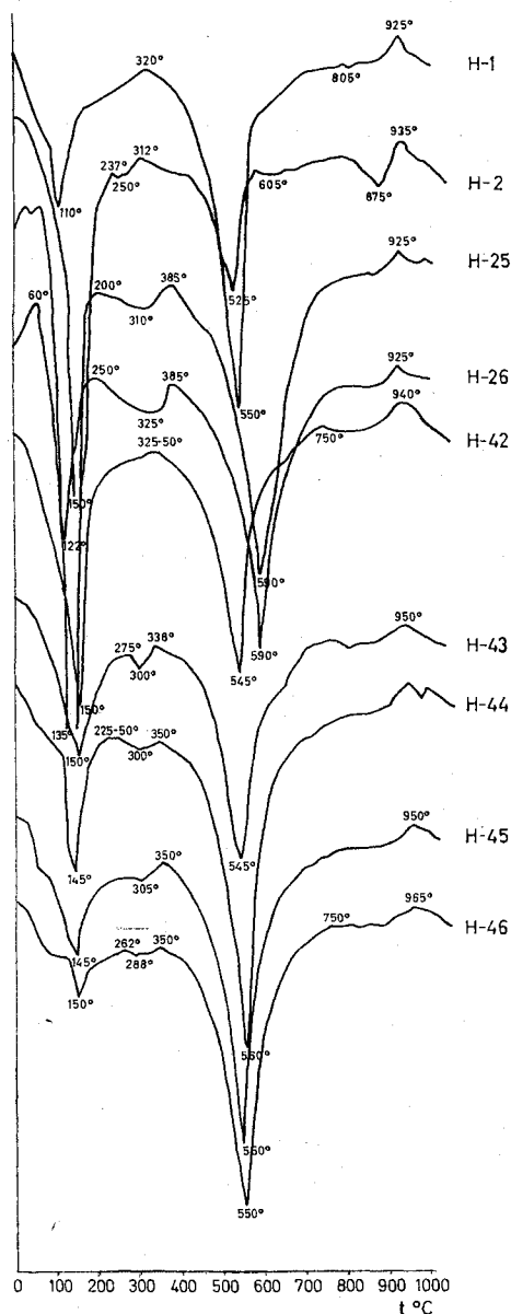
FIG. 6.—Curvas de análisis térmico diferencial de las muestras procedentes de yacimientos sobre pizarras.
