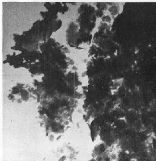
FIG. 8.— Microfotografías electrónicas de la muestra H-5. Microlaminillas atípicas de illita-montmorillonita y haloisita heterométrica frecuente.
