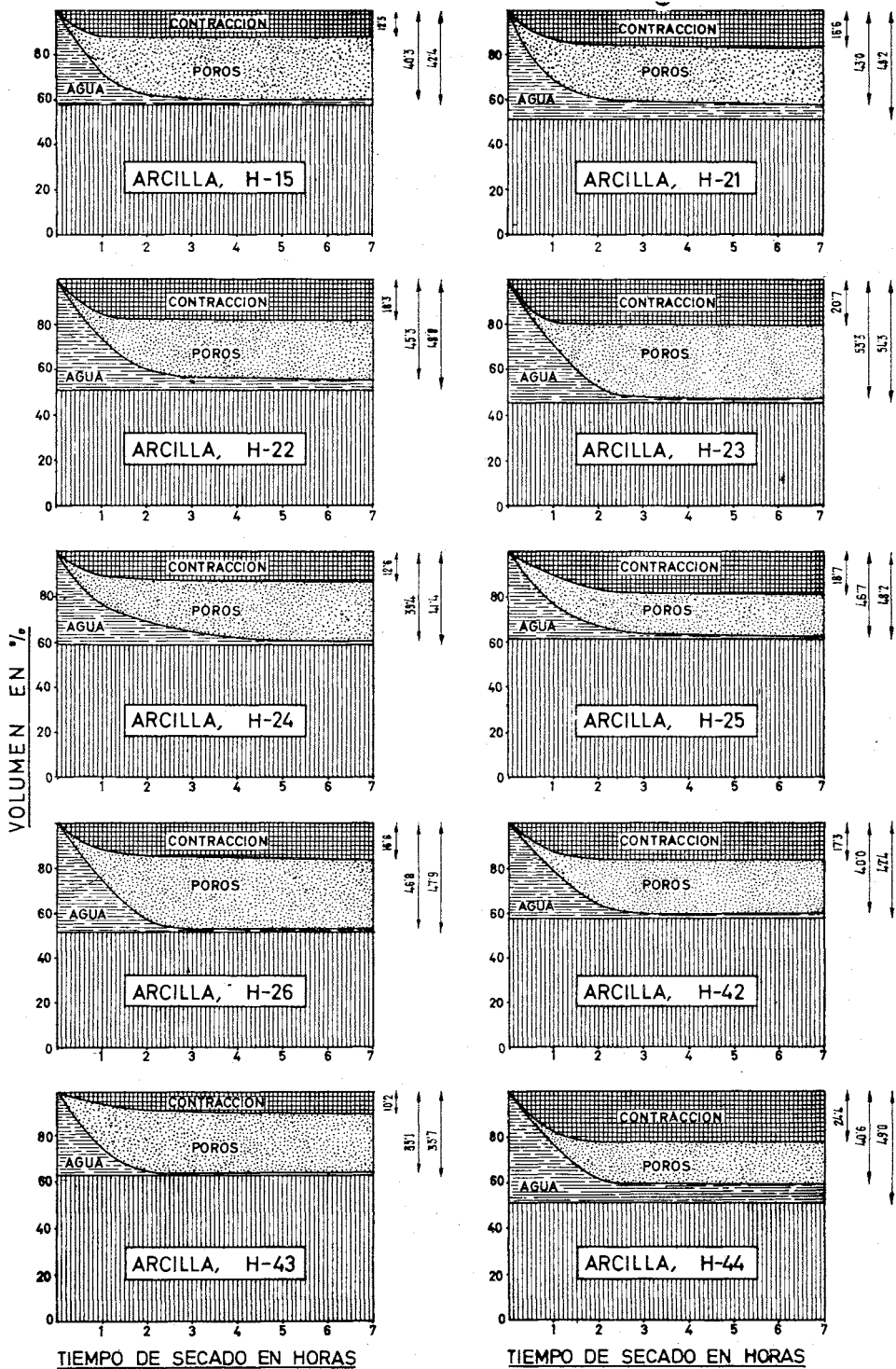
Fig 11.—Diagramas de secado a 50°C de las muestras H-15 a la H-44.
