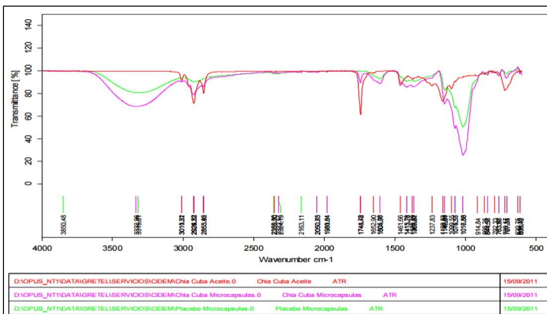
Figura 15: 2. Espectros infrarrojos del aceite sin microencapsular (Rojo), microencapsulado (Morado) y de los polímeros (Verde) (López y cols., 2015).
