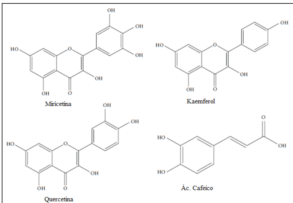
Figura 14: moléculas orgánicas de los antioxidantes fenólicos presentes en extractos de semilla de Chía (Mohd Ali y cols., 2012).
