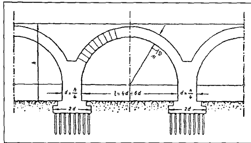
Figura 1. Traza de un puente según las reglas de Alberti (Straub, 1992)
