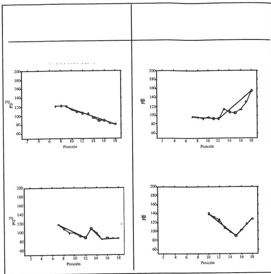
Figura 3: Clasificación de los patrones finales del español definidos en Estruch-Garrido (1995)
