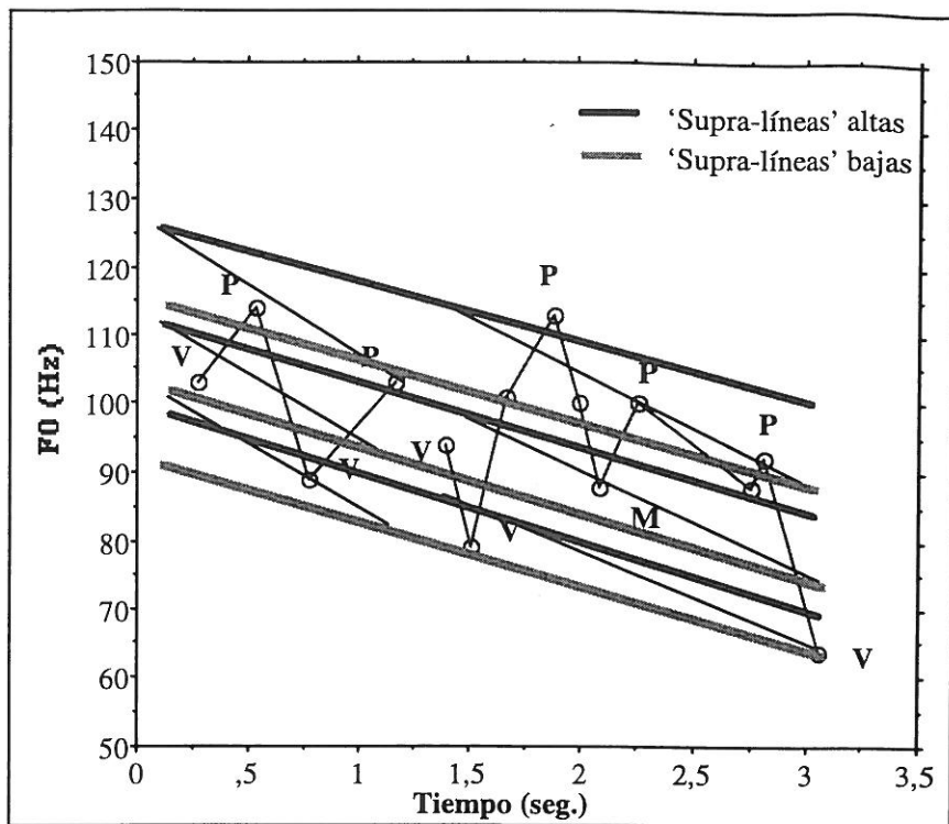
Figura 6. 'Supra-líneas' superior e inferior calculadas para los grupos fónicos del enunciado 'La organización terrorista ha protagonizado en lo que va de año una escalada de atentados en los que han perdido la vida quince personas', pronunciado por un locutor masculino.
