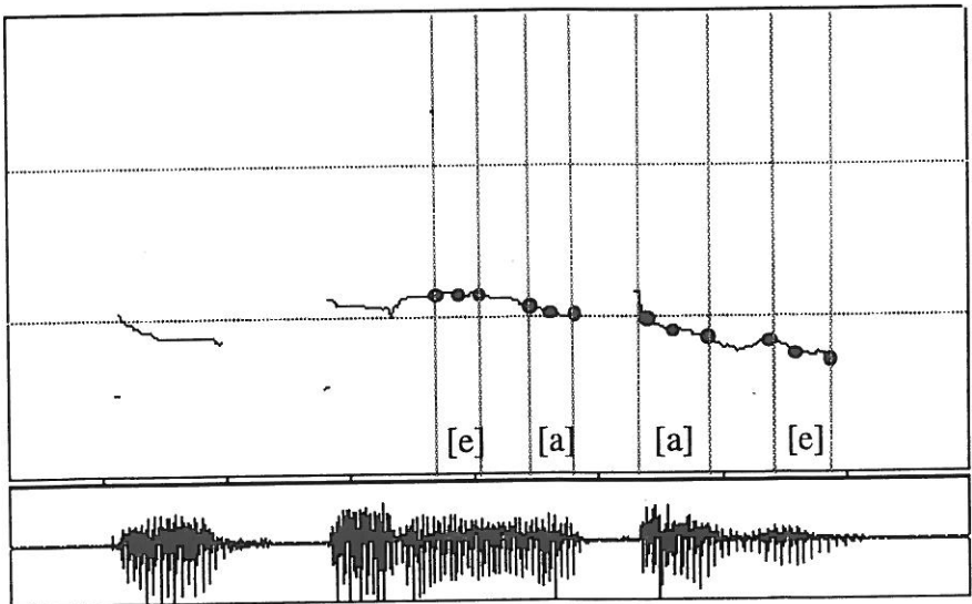
Figura 1. Curva melódica correspondiente al enunciado 'Te espero en la calle'. Las líneas verticales indican los límites de las vocales del grupo acentual 'en la calle'. Los puntos de cada vocal en que se tomaron los valores de F0 están marcados con círculos negros.
