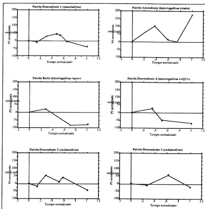
Figura 4: Patrones melódicos de la frase simple del catalán definidos en Estruch et al. (1994)
