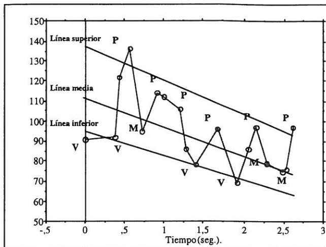
Figura 5. Líneas superior, media e inferior correspondientes al enunciado 'La organización terrorista ha protagonizado en lo que va de año', pronunciado por un locutor masculino.
