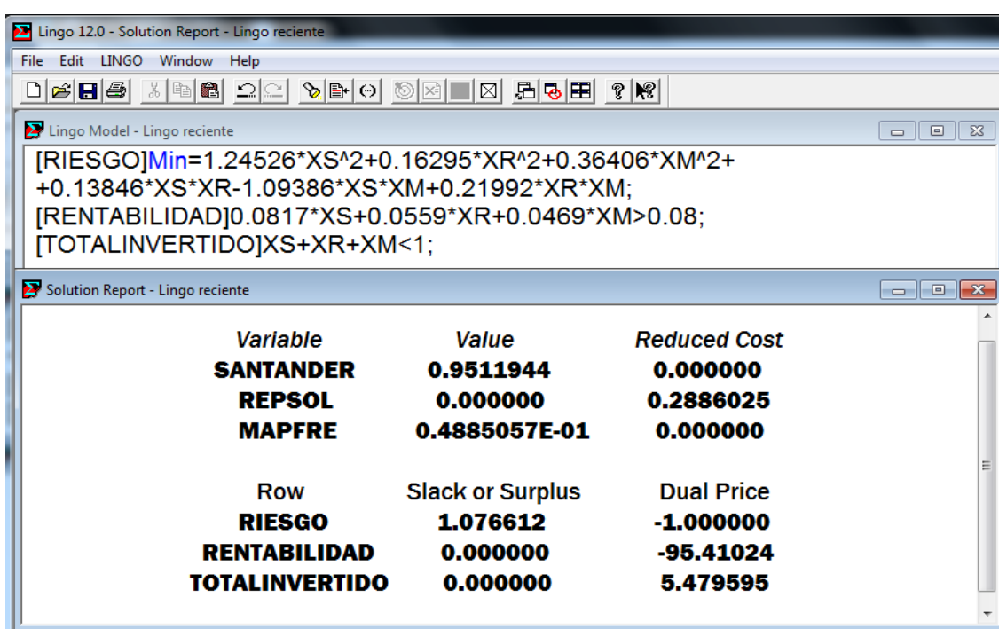
Figura 5.1. Solución del problema para una rentabilidad mínima del 8 % proporcionada por LINGO
