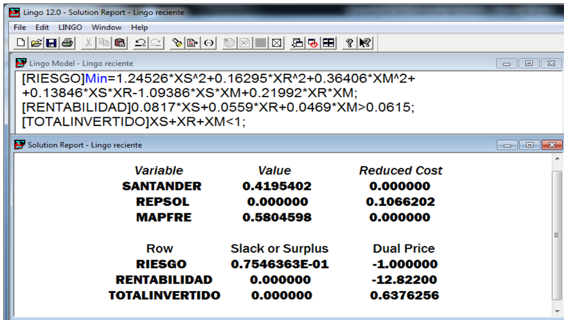
Figura 5.2. Solución del problema para una rentabilidad mínima del 6,15 % proporcionada por LINGO
