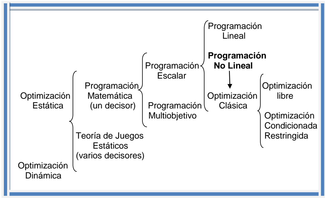
Esquema 1.1. Clasificación de la Optimización Matemática
