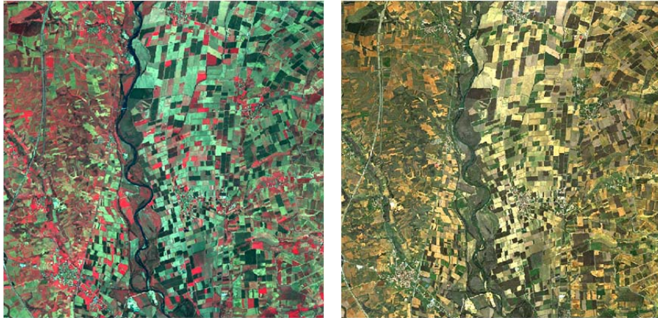
Figura 1. Compuesto RGB de una imagen Landsat8 en falso Falso Color infrarrojo (izquierda) y en color natural (derecha).
