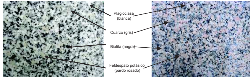
Figura 6. Ejemplo de descripción "de visu" de un granito (entre los nº 23-25 de la calle).
