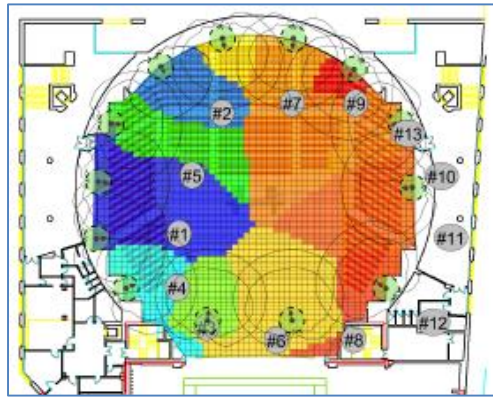
Figura 4-29 Zona que abarca cada AP en el Patio de Butacas
