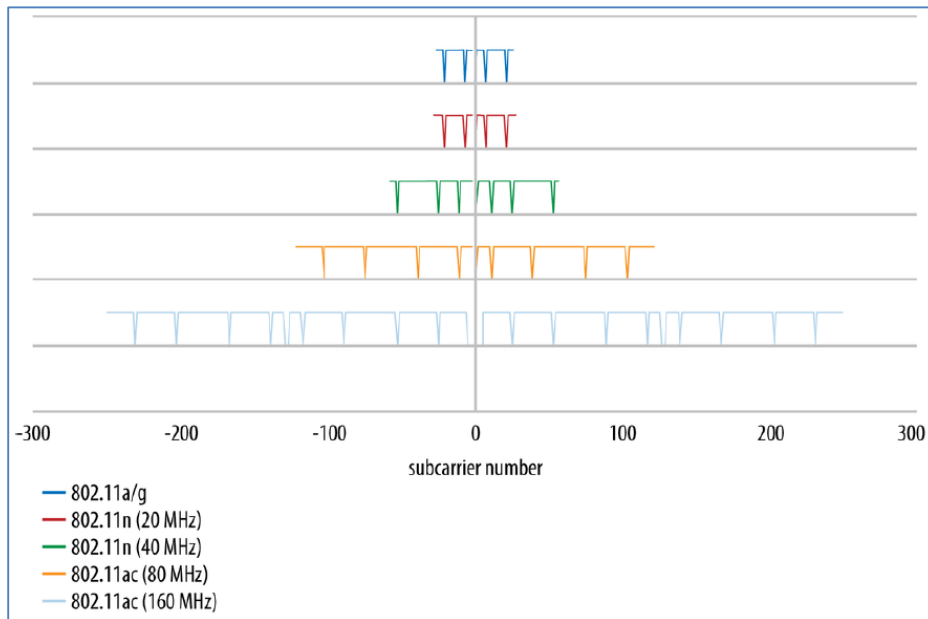
Figura 3-1 Diseño de los canales
