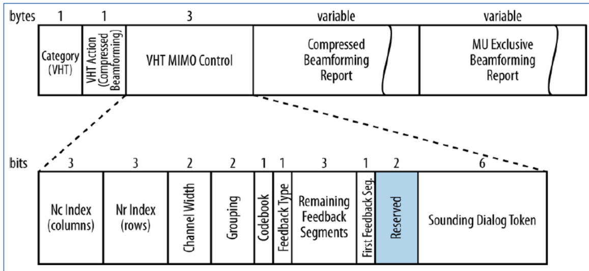
Figura 5-12 Trama de acción comprimida
