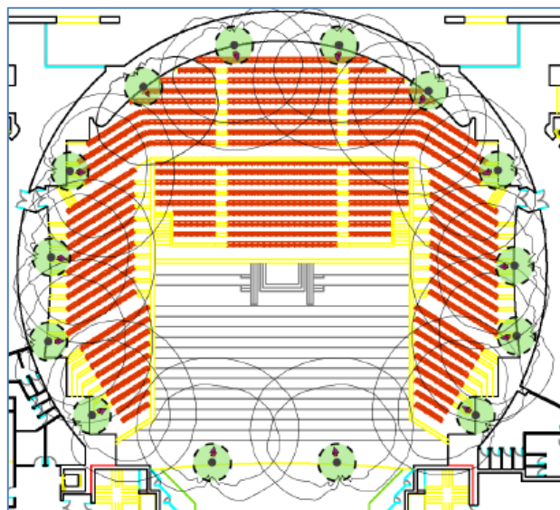
Figura 4-19 Posición de los APs en la zona principal
