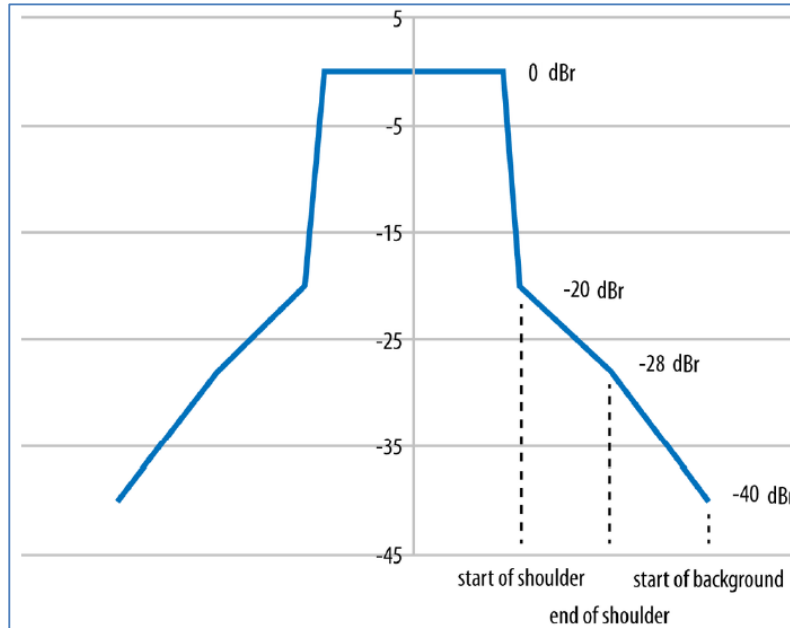
Figura 3-2 Máscara espectral
