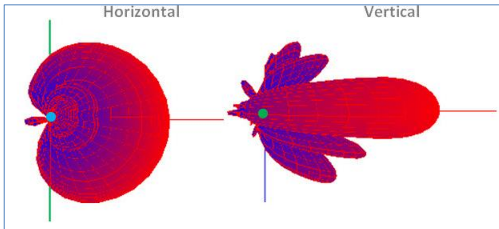
Figura 4-3 Diagramas de radiación horizontal y vertical
