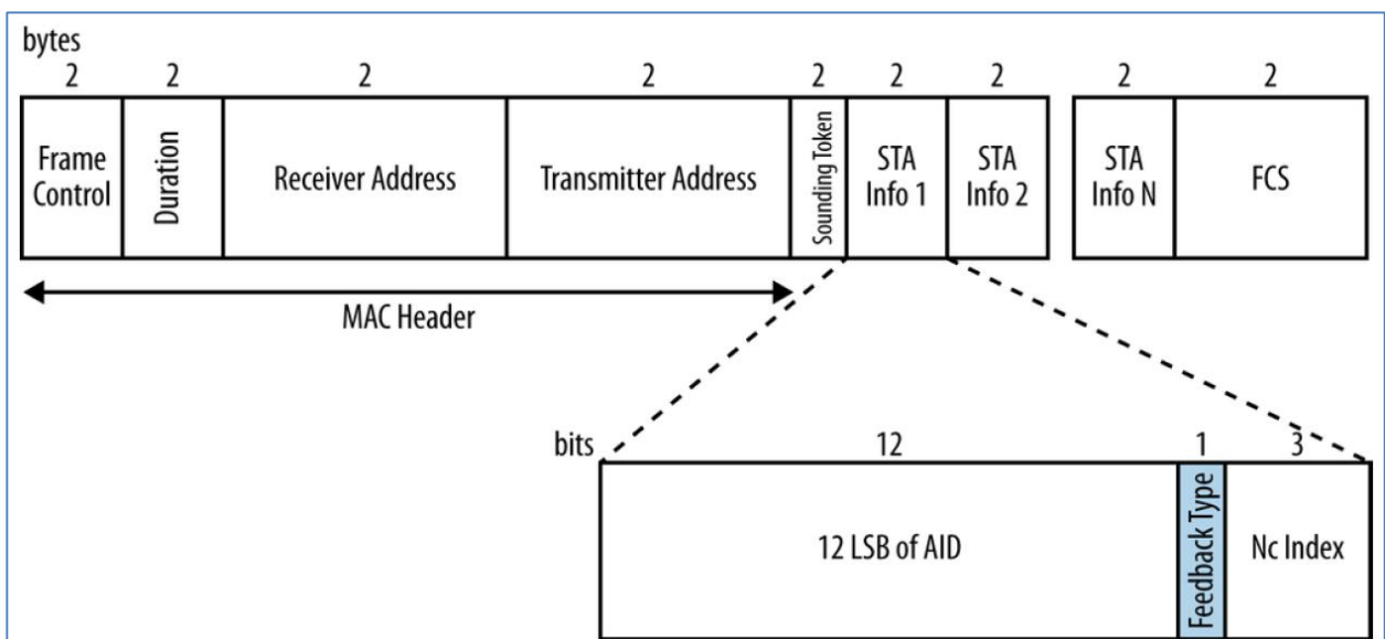
Figura 5-11 Trama de anuncio NDP Multiusuario
