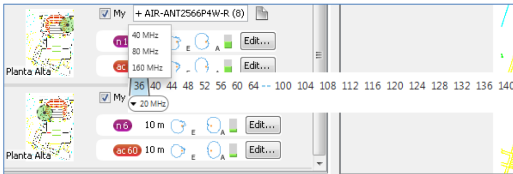
Figura 4-23 Cambio de canal y ancho de banda 802.11ac
