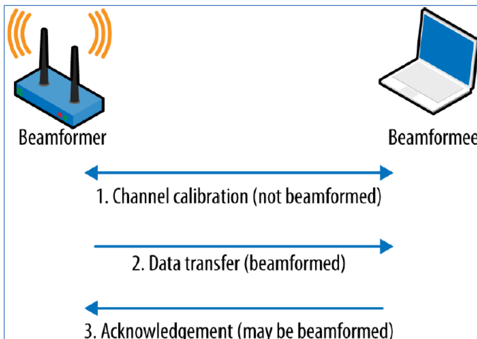
Figura 5-2 Proceso de beamforming simplificado
