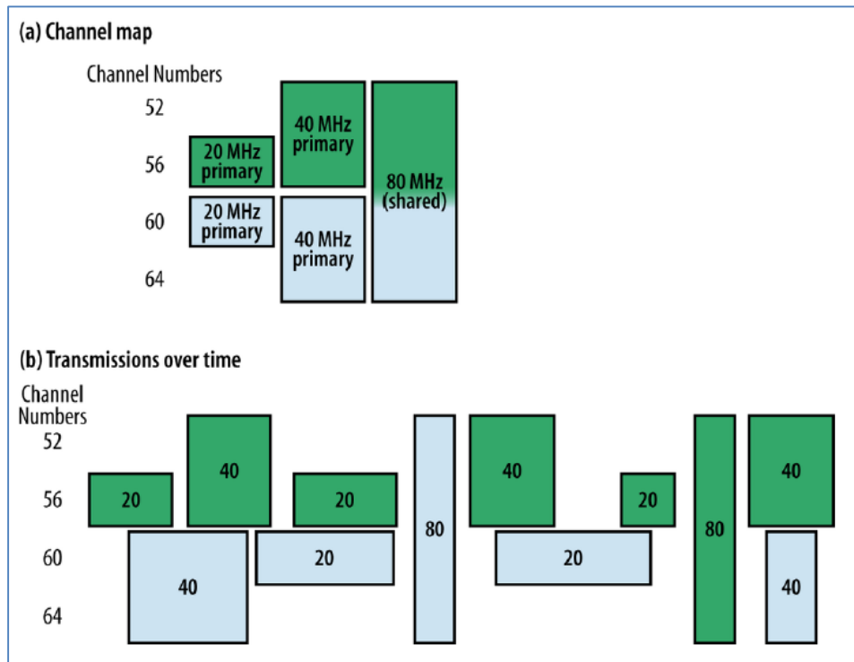
Figura 3-12 Canal compartido por varias redes
