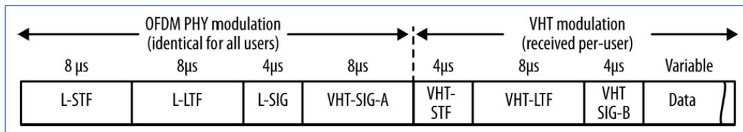
Figura 3-6 Trama PHY 802.11ac
