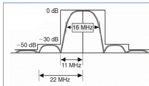
Figura 2-11 Máscara espectral
