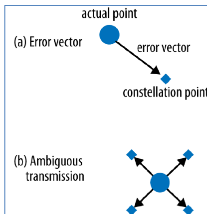
Figura 3-5 Vector de error
