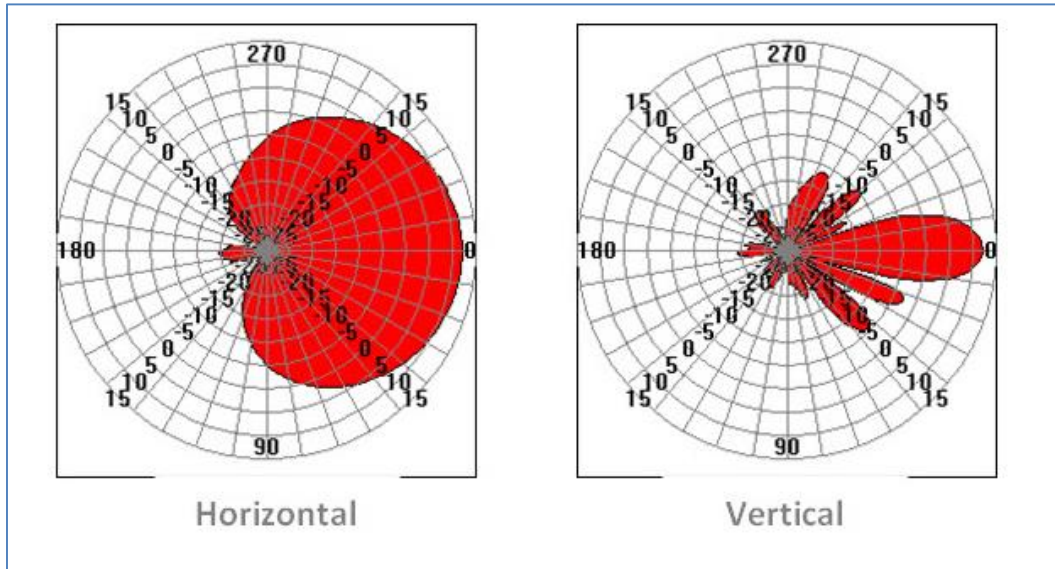
Figura 4-4 Diagramas de radiación con escalas
