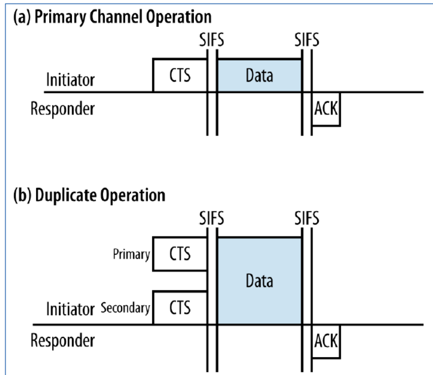
Figura 3-10 Proceso de acceso al canal
