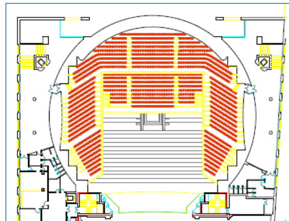
Figura 4-12 Plano planta superior
