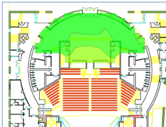
Figura 4-32 Nivel de señal en Sala de Prensa
