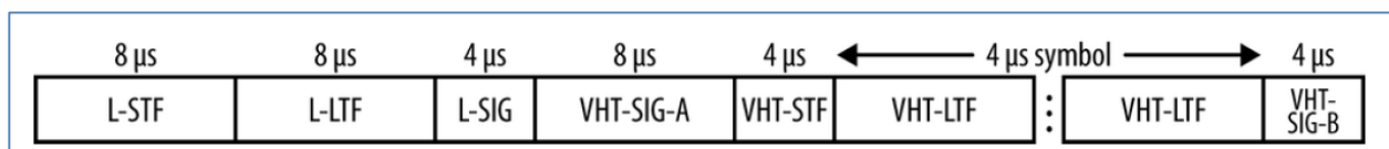
Figura 5-8 Formato trama NDP
