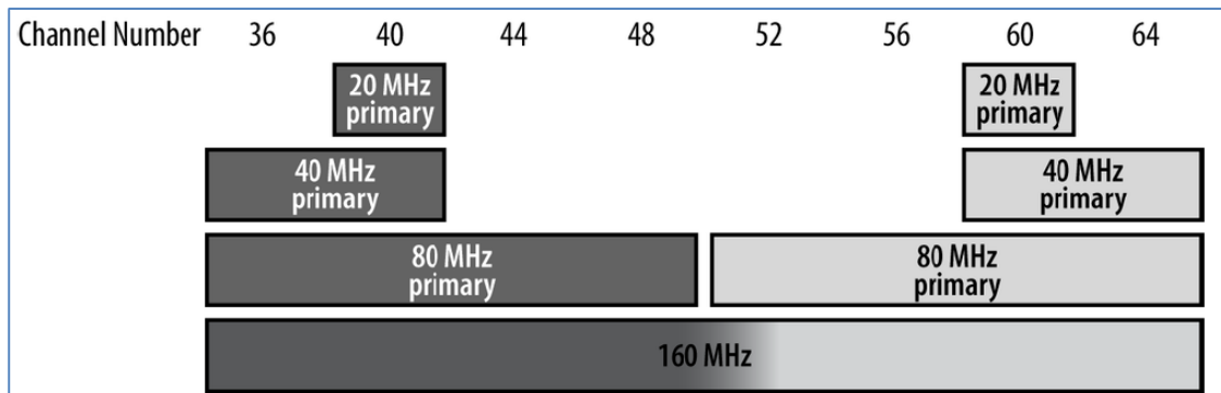
Figura 3-9 Coexistencia de varias redes en una misma frecuencia
