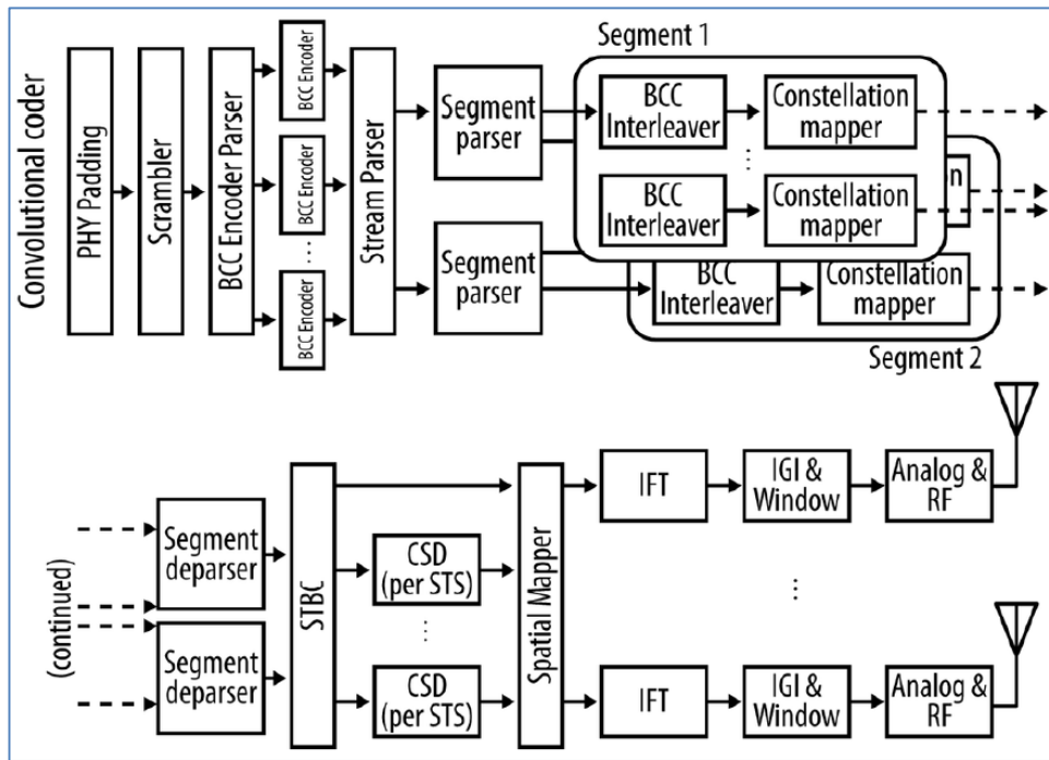
Figura 3-7 Diagrama de bloques para transmisión y para recepción
