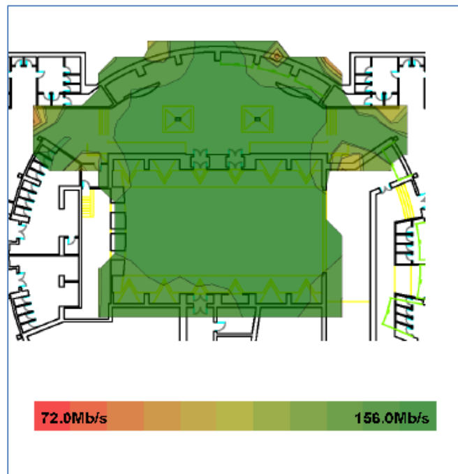
Figura 4-35 Ancho de banda en zona catering
