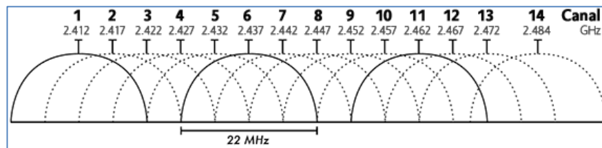
Figura 2-5 Canales disponibles según la nota UN-85
