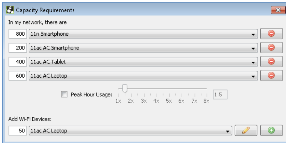
Figura 4-15 Requisitos de conectividad para patio de butacas
