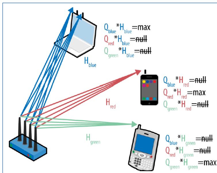
Figura 5-16 Interferencia interusuario
