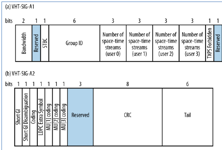
Figura 5-15 Formato de la trama de acción para el caso multiusuario
