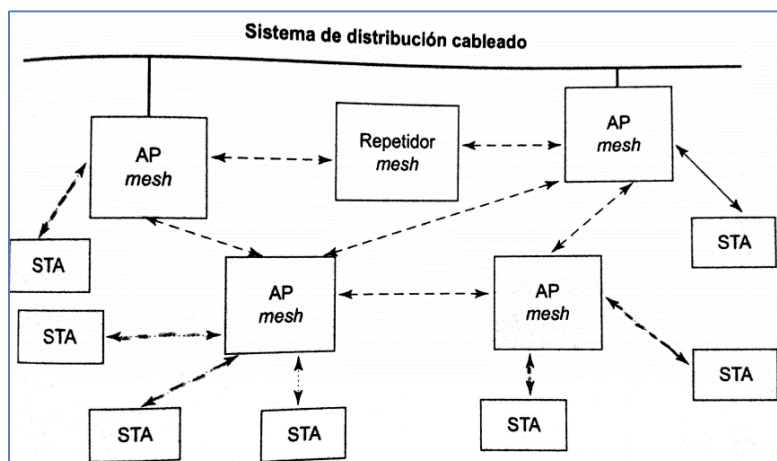
Figura 2-3 Redes en malla
