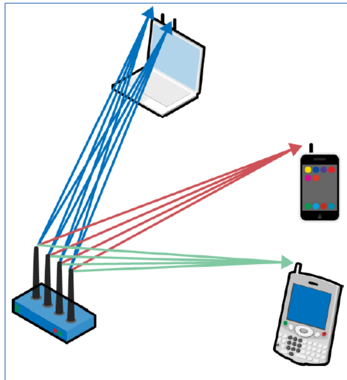
Figura 5-14 Distintas rutas MIMO multiusuario
