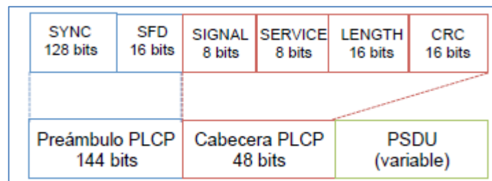
Figura 2-7 Formato trama señal WiFi
