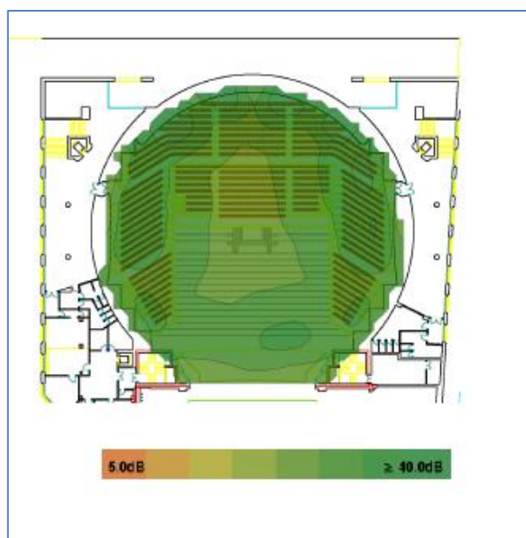
Figura 4-28 Valor de SNR en el Patio de Butacas
