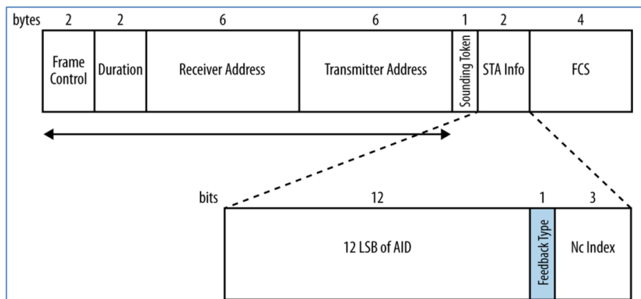
Figura 5-7 Formato trama de anuncio NDP
