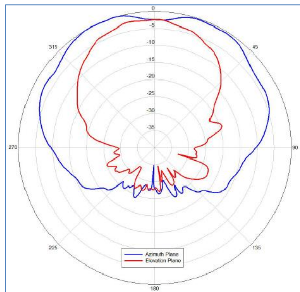
Figura 4-9 Diagrama de radiación banda 5 GHz
