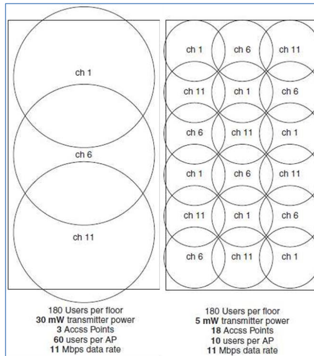
Figura 4-10 Diferencia entre entorno típico y entorno de alta densidad
