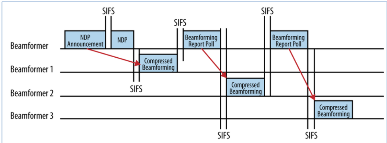
Figura 5-10 Procedimiento de calibración del canal
