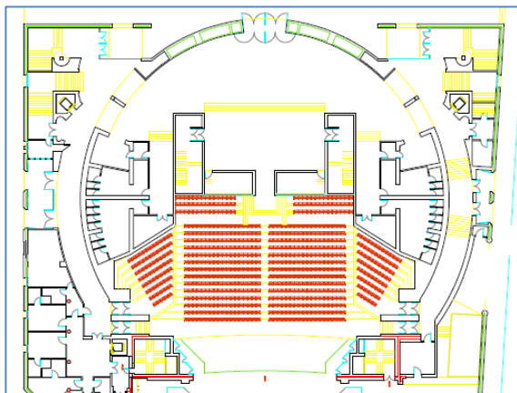
Figura 4-11 Plano planta inferior
