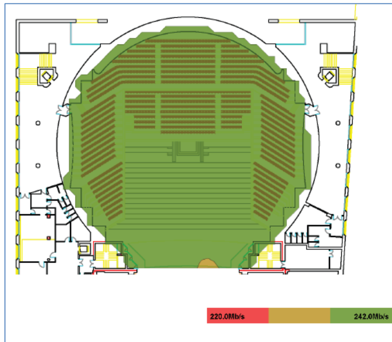
Figura 4-27 Ancho de banda en el Patio de Butacas
