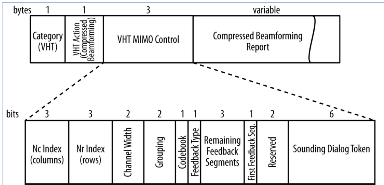
Figura 5-9 Formato de la de la matriz de acción
