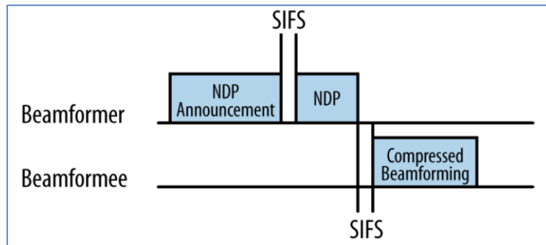
Figura 5-6 Calibración del canal
