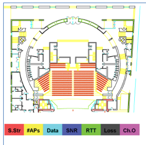
Figura 4-30 Salud de la red
