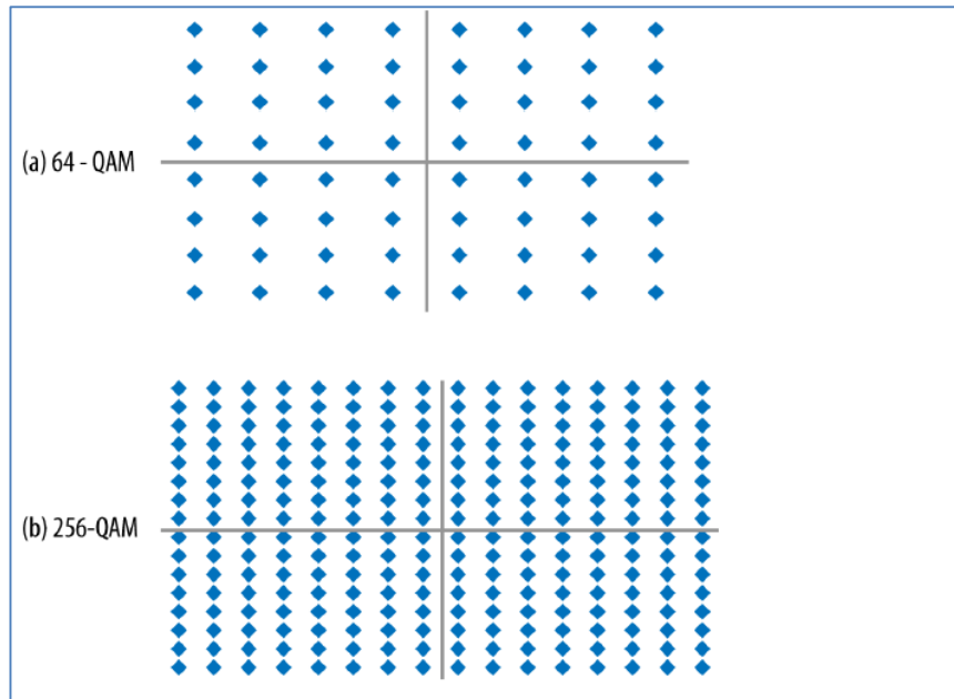
Figura 3-4 Comparación de las modulaciones 64-QAM y 256-QAM
