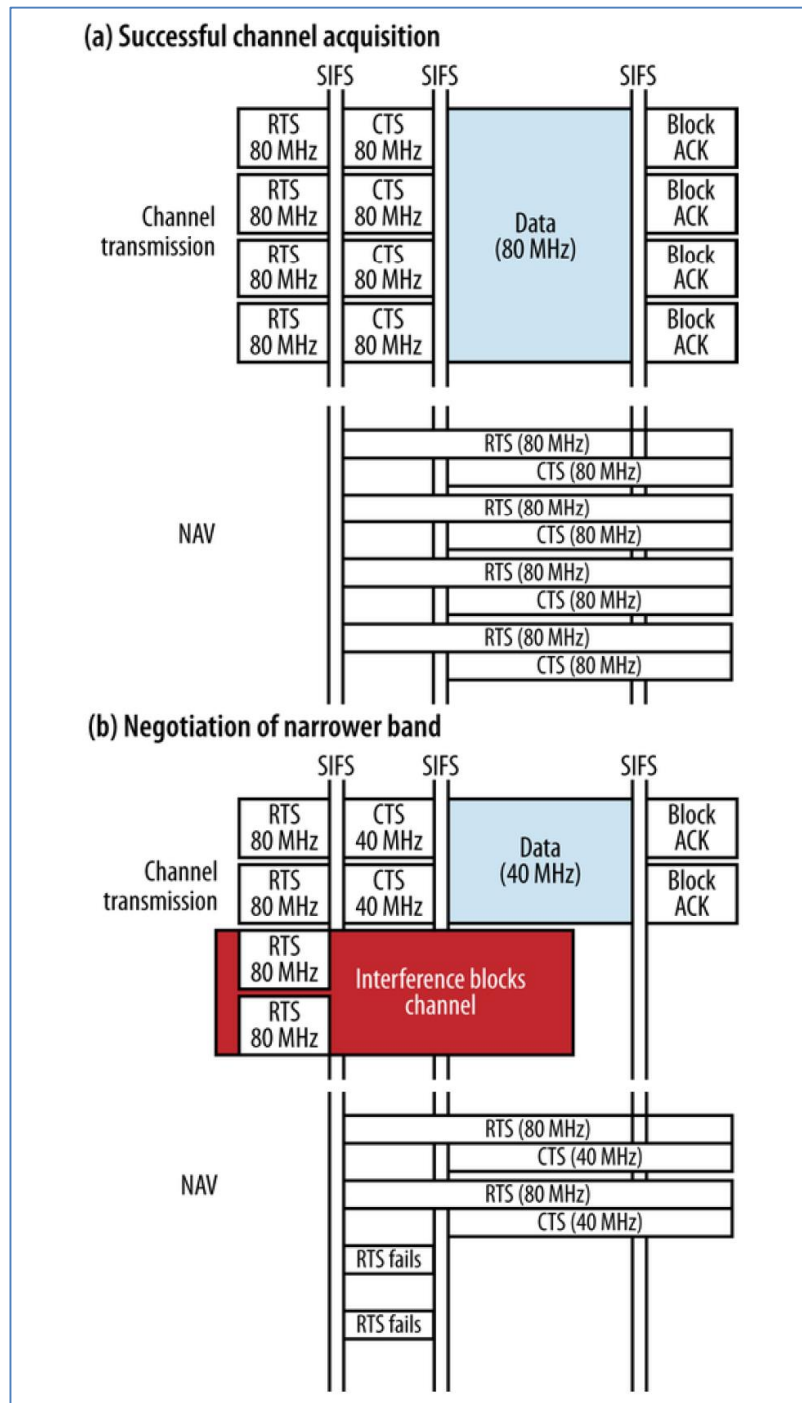
Figura 3-11 RTS y CTS trabajando conjuntamente
