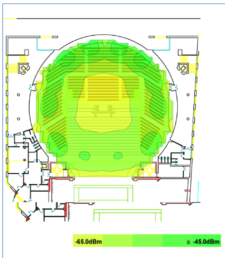
Figura 4-26 Nivel de señal en el Patio de Butacas
