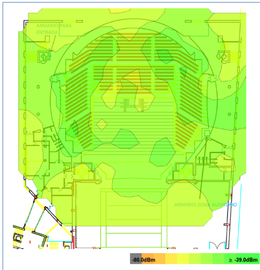
Figura 4-37 Resultado cobertura Site Survey
