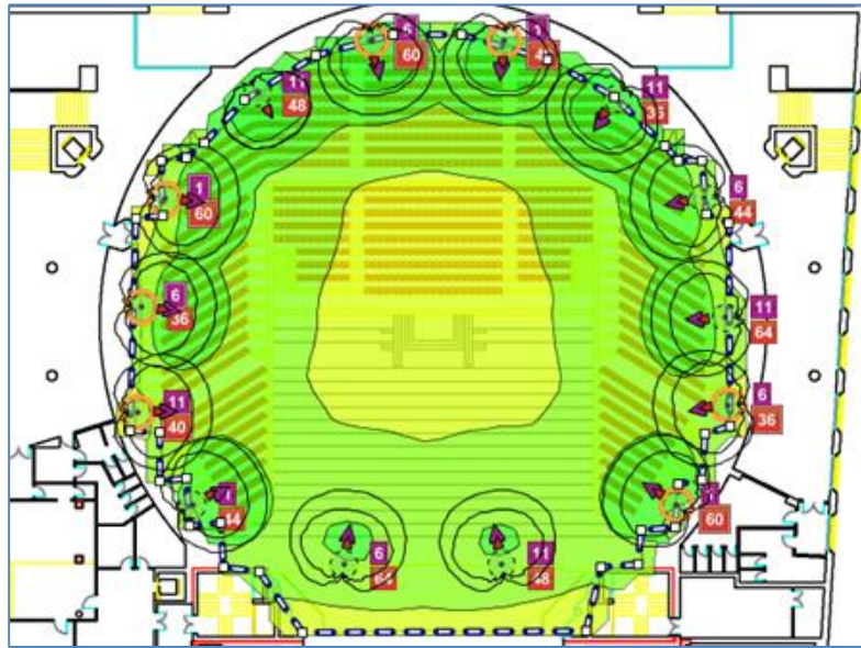
Figura 4-25 Distribución de los canales en ambas bandas
