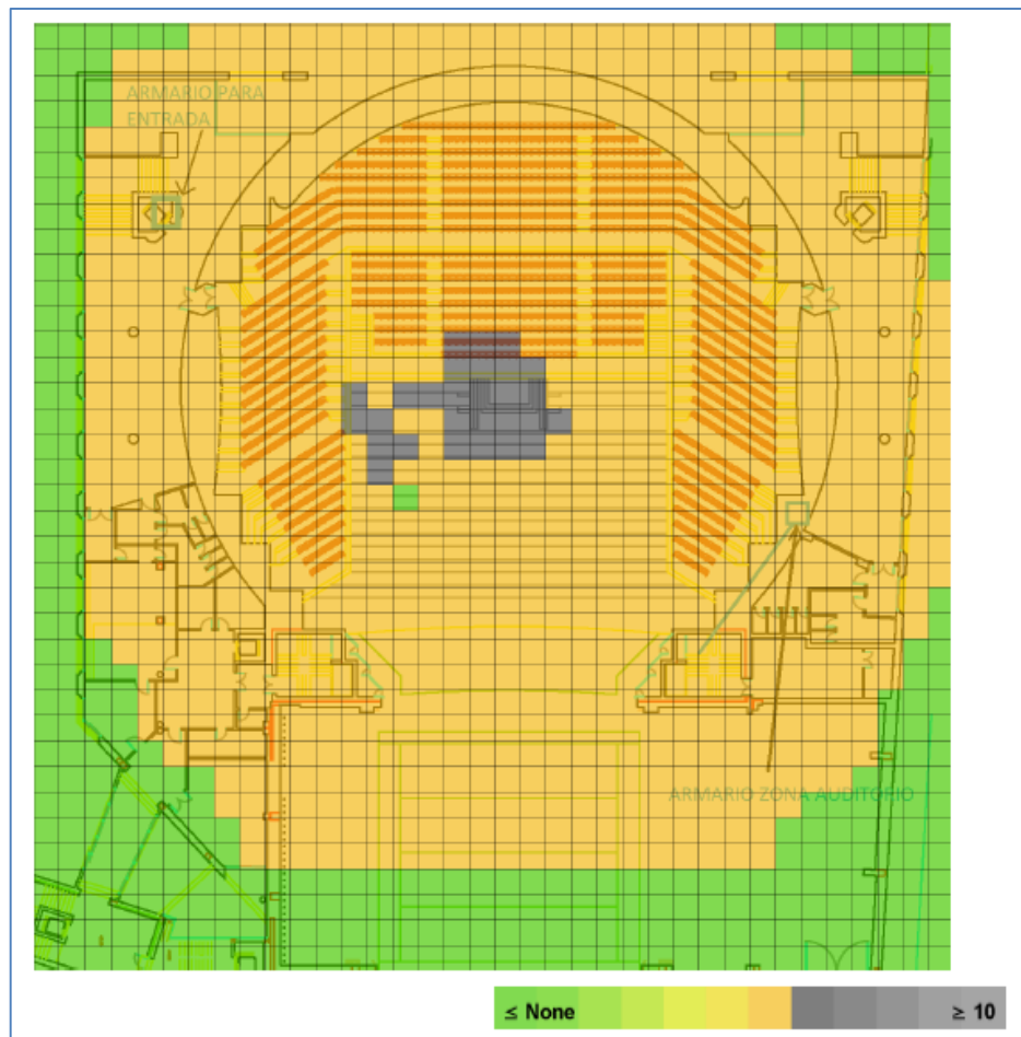
Figura 4-38 Solapamiento de canales Site Survey
