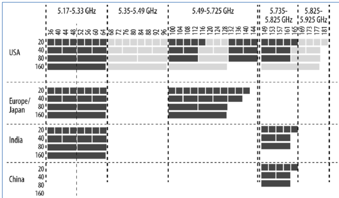
Figura 3-3 Canales disponibles en cada región
