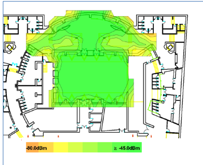
Figura 4-36 Cobertura en zona de catering
