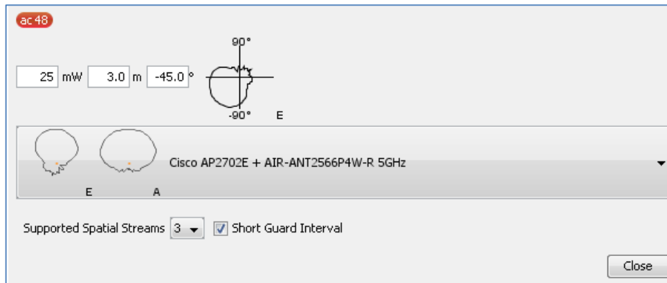
Figura 4-22 Parámetros configurables de la antena
