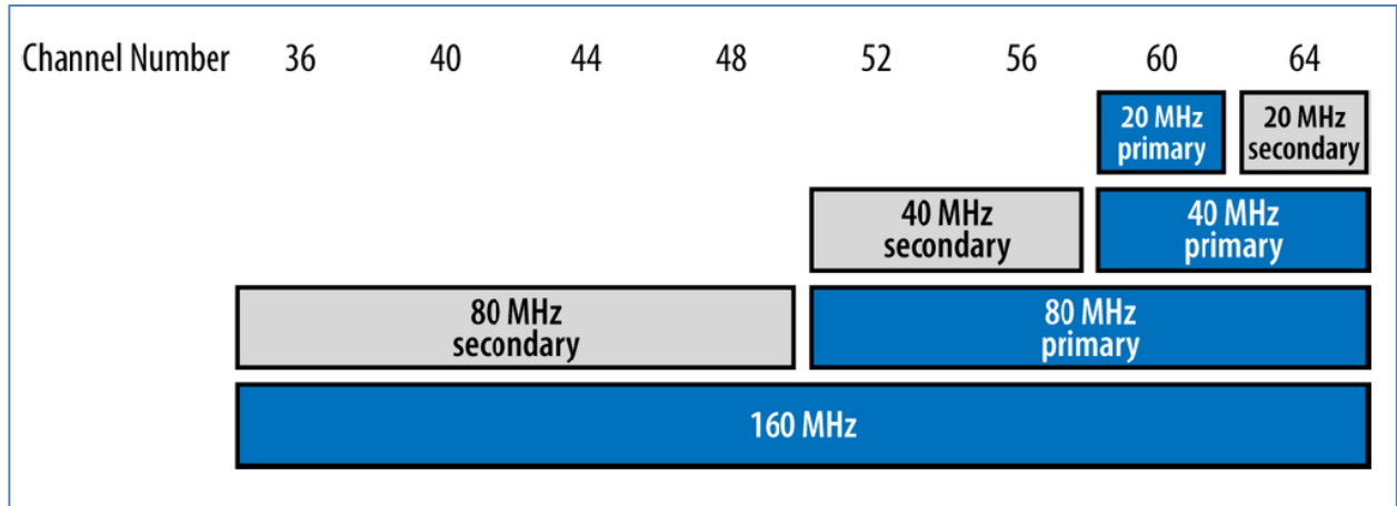
Figura 3-8 Canales primarios y secundarios
