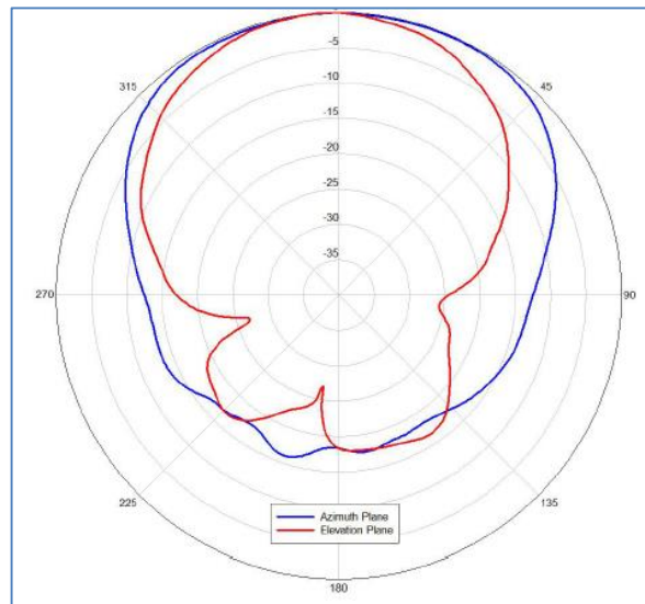
Figura 4-8 Diagramas de radiación banda 2,4 GHz
