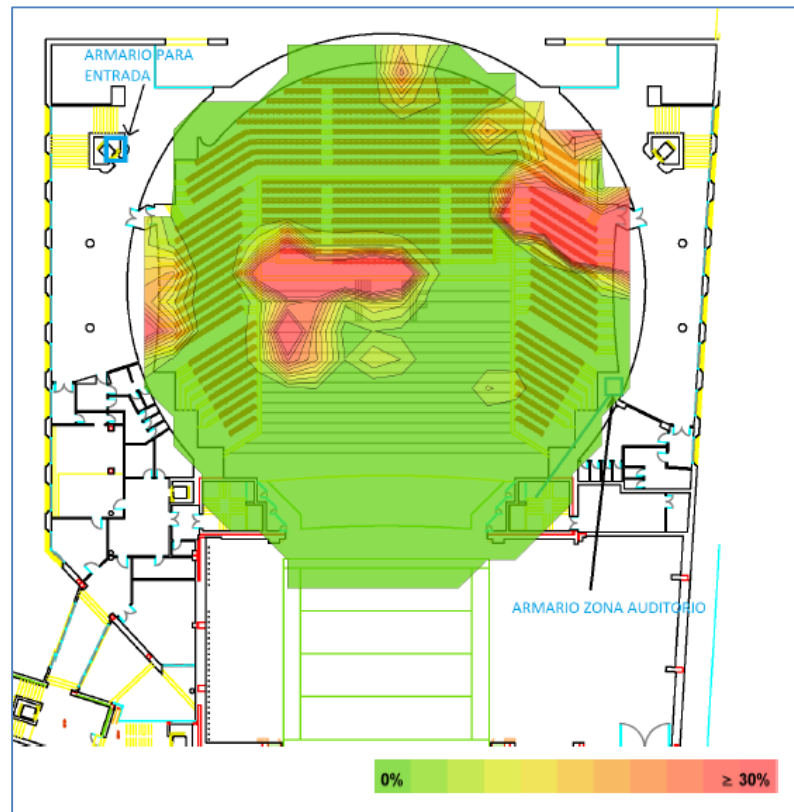
Figura 4-39 Pérdida de paquetes
