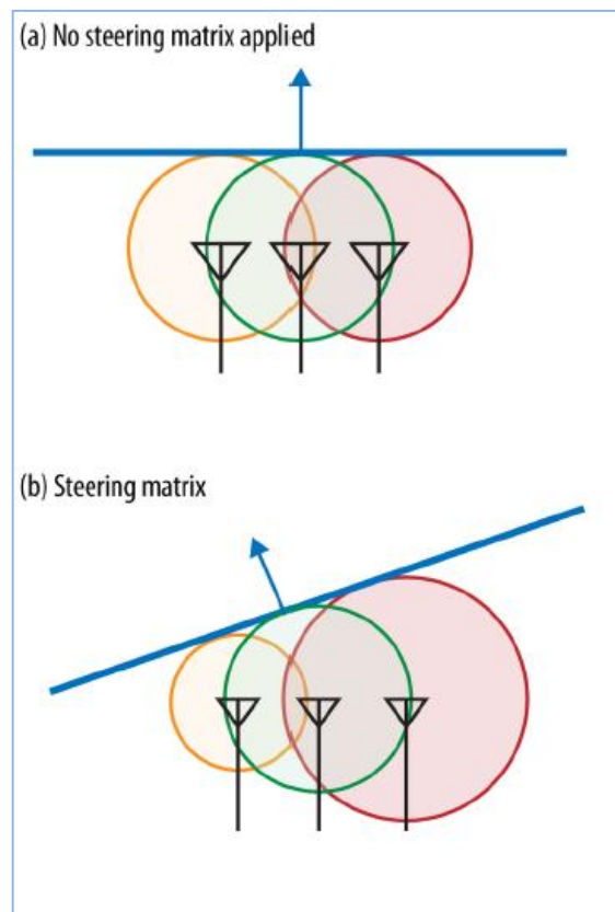
Figura 5-3 Desfase entre arrays
