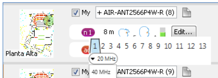
Figura 4-24 Cambio de canal y ancho de banda 802.11n
