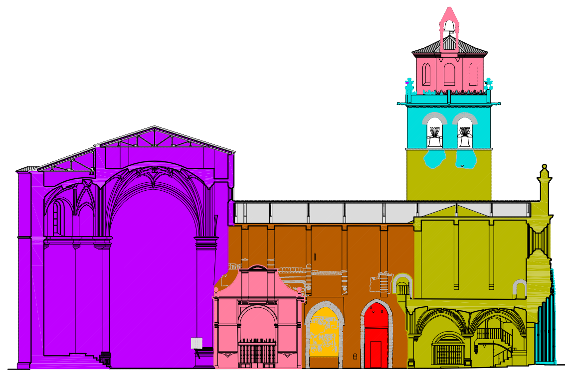
SECCIÓN BB'
