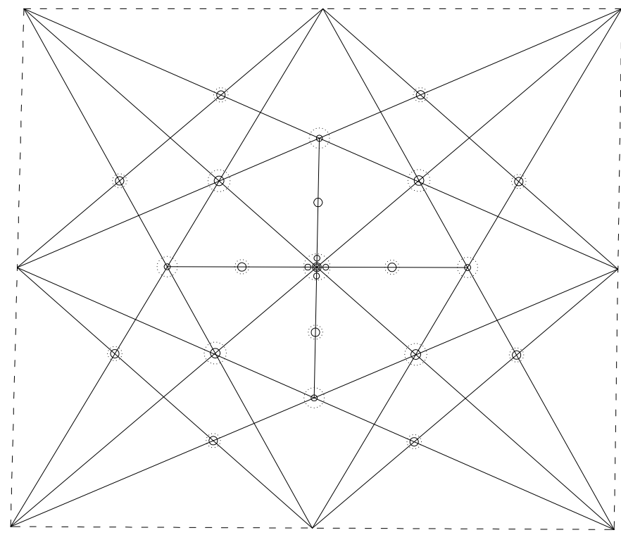
DESARROLLO DE LA BÓVEDA DEL CRUCERO
