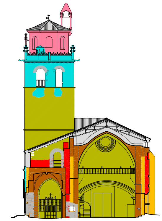
SECCIÓN CC'
