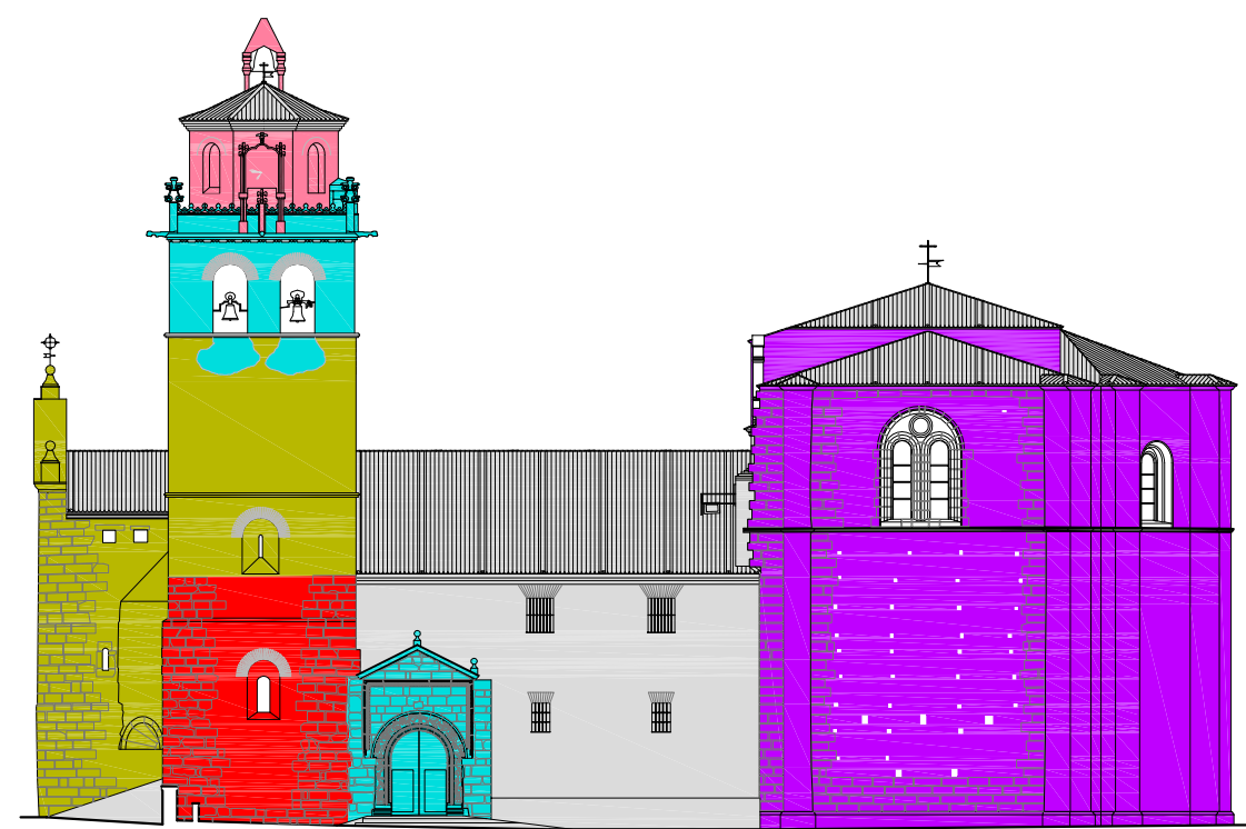
ALZADO SUR
