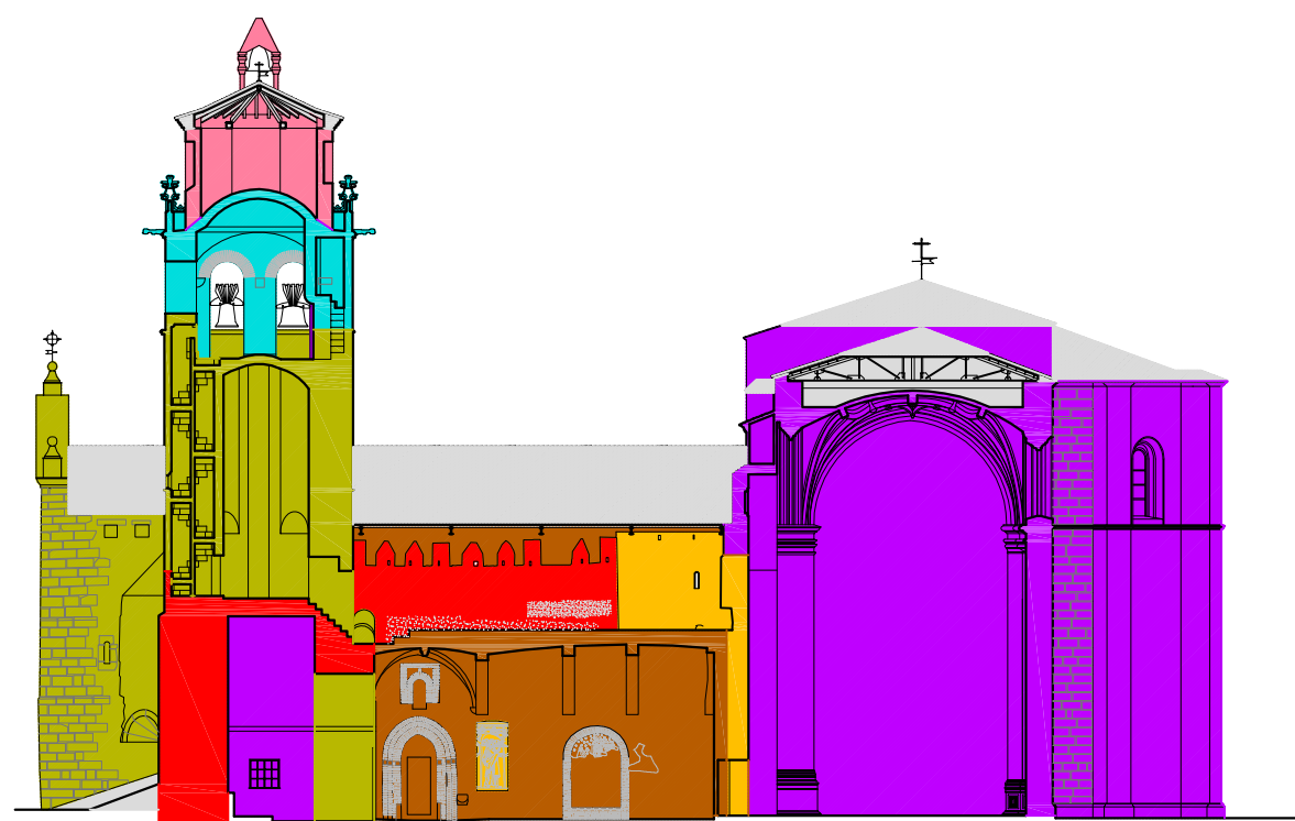
SECCIÓN EE'
