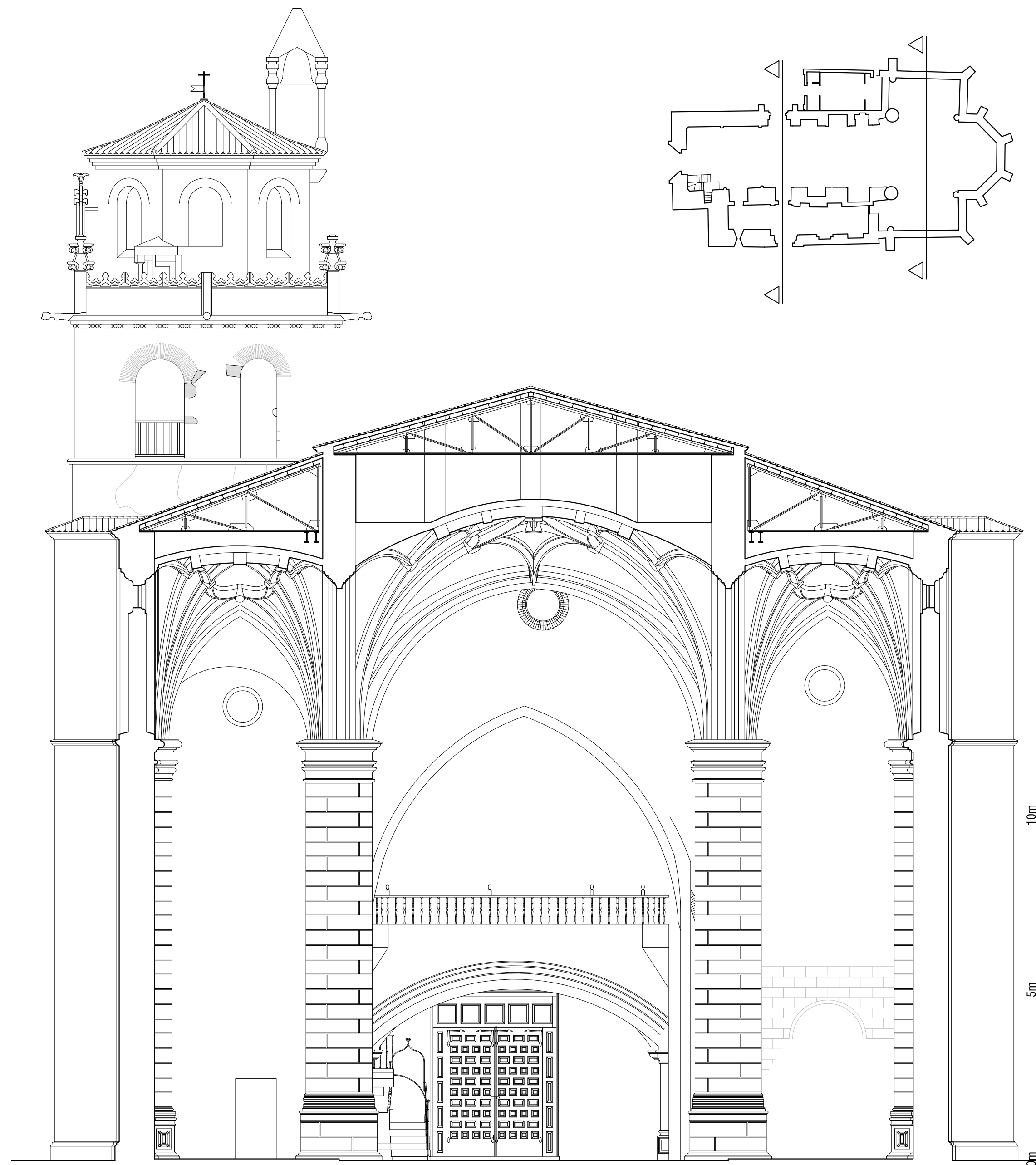
SECCIÓN DD'
