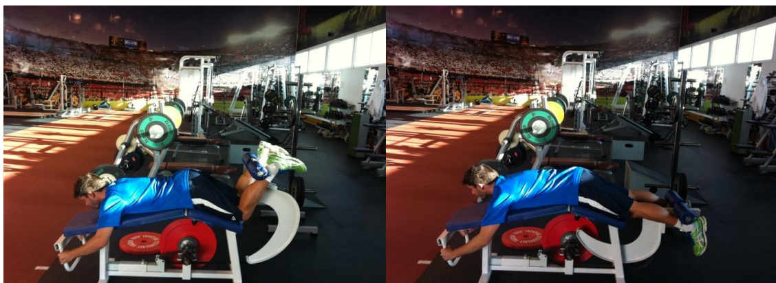
Figura 1. Dispositivo YoYo™ para leg curl y ejercicio desarrollado en el estudio.
