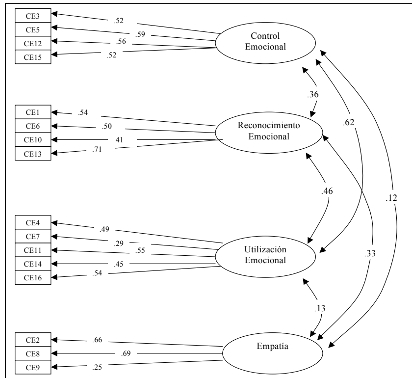
Figura 2. Parámetros estimados para el modelo reespecificado.
