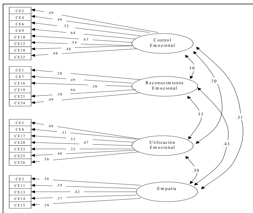
Figura1. Parámetros estimados para el modelo original
