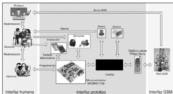
Figura 4. Estructura detallada del sistema de control.
