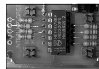
Figura 9. Fotografía de la lógica OR del circuito de adaptación
