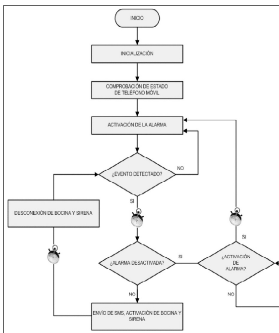
Figura 5. Diagrama de Flujo del Sistema de Control.
