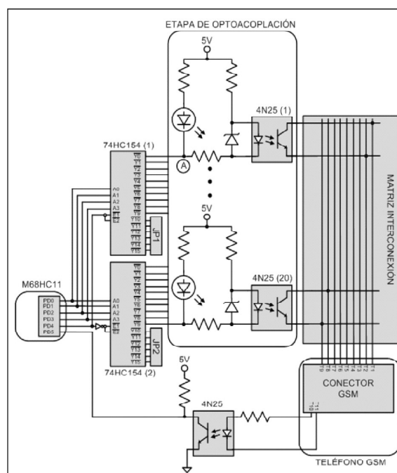
Figura 8. Interfaz Microcontrolador-Teléfono Móvil
