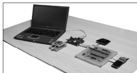
Figura 3. Fotografía del banco de pruebas del sistema.
