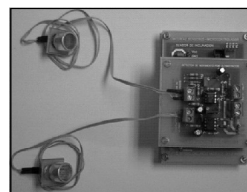
Figura 8. Fotografía del sensor de intrusismo
